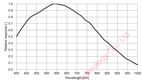
MV-CA016-10UM 量子效率
