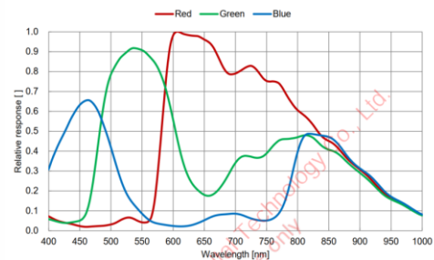
MV-CA016-10UC 量子效率
