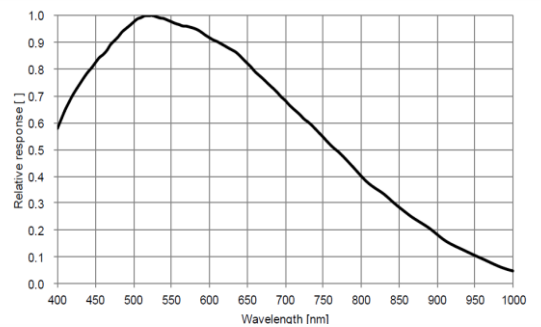
MV-CA023-10UM 量子效率
