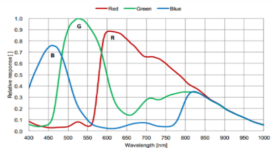
MV-CA023-10UC 量子效率
