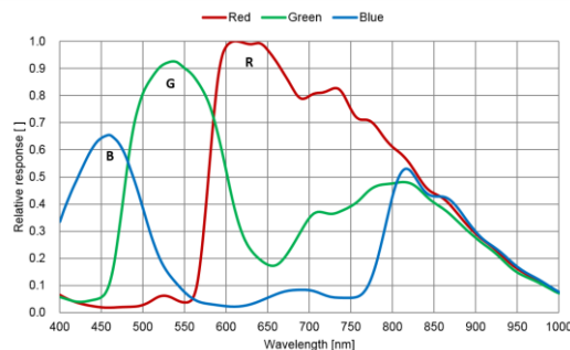
MV-CA050-10GC 量子效率
