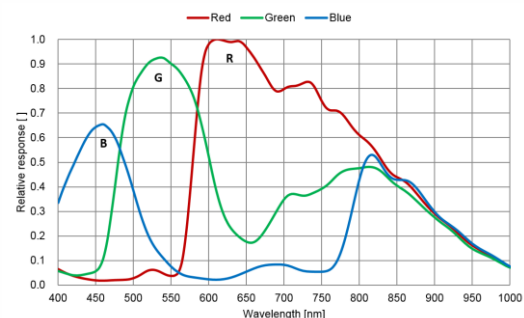
MV-CA050-11UC 量子效率
