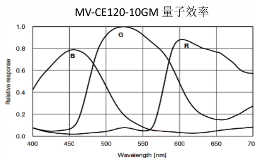
MV-CE120-10GC 量子效率
