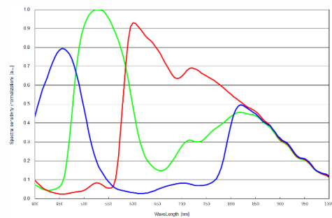
MV-CE200-10UC 量子效率
