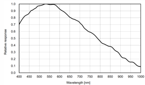
MV-CE200-10UM 量子效率
