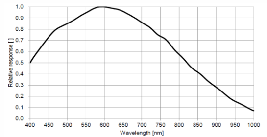
MV-CU004-10GM 响应曲线
