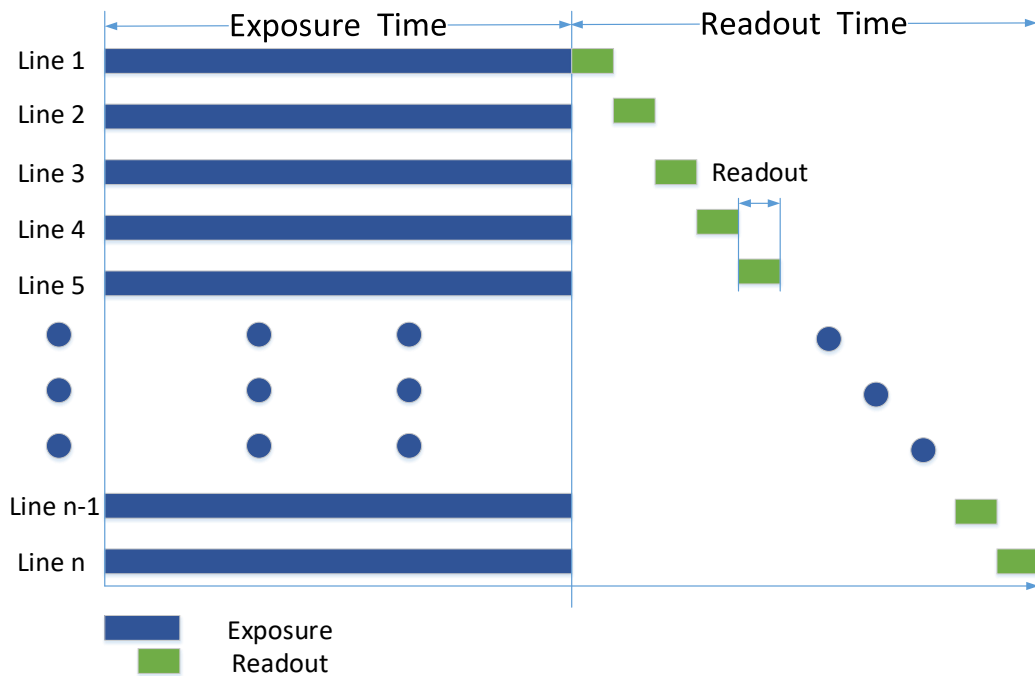
图9-1 全局快门
