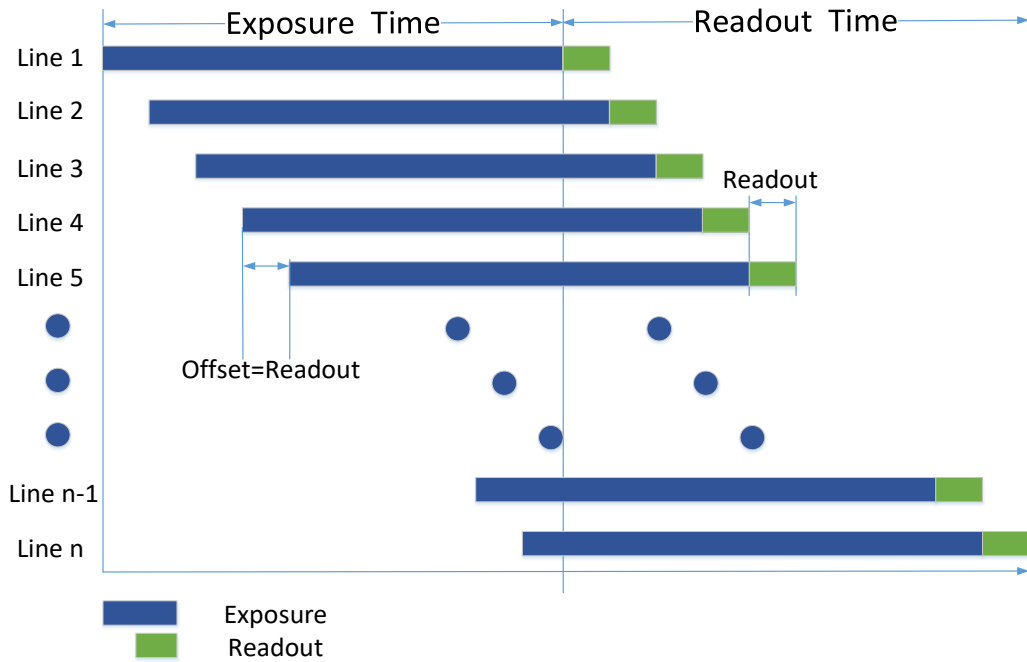
图9-2 卷帘快门
