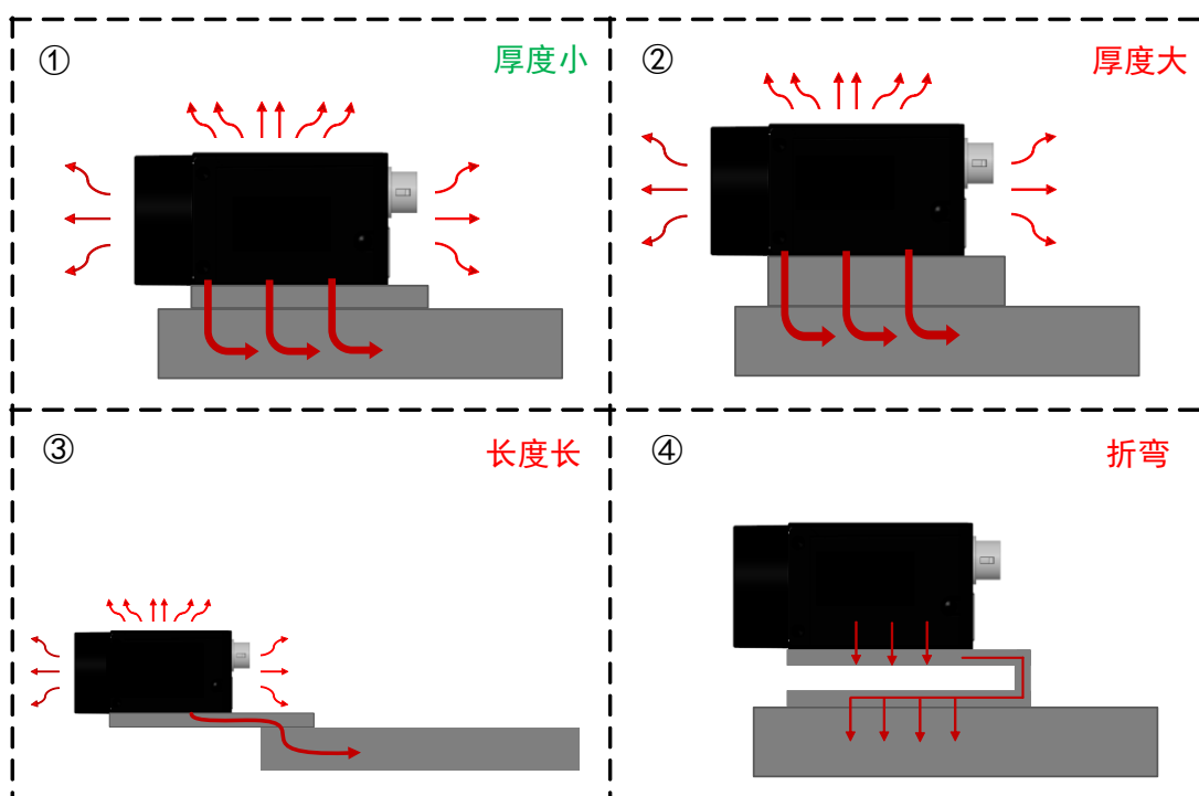
图5-4 不同安装方式的导热路径
