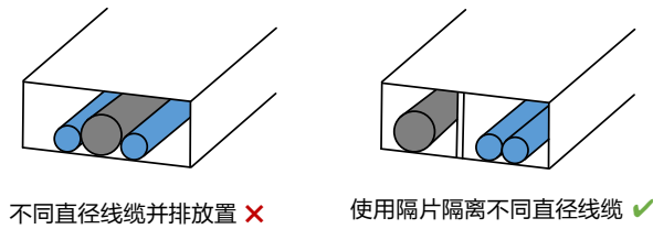
图4-11 隔片分离隔离
