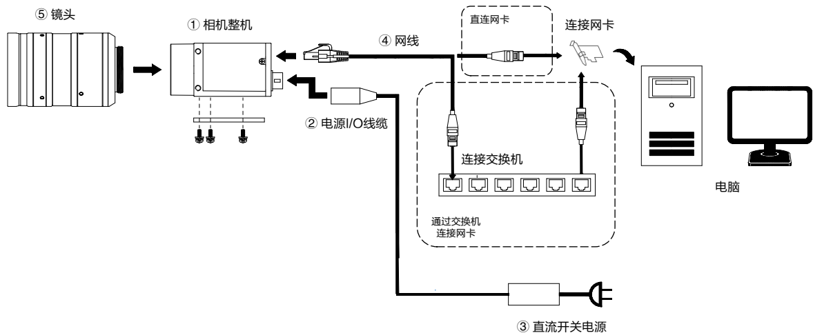
图6-2 整机连接
