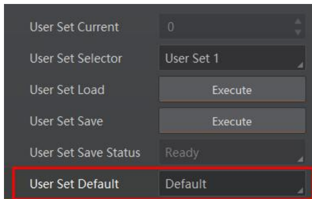
图11-40 设置默认启动参数
