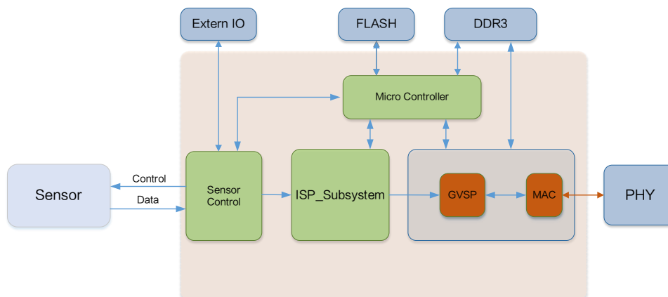
图3-1 工作原理
