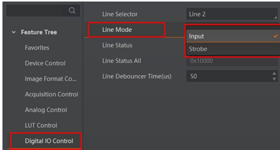
图8-5 Line 2 设置为输入信号
