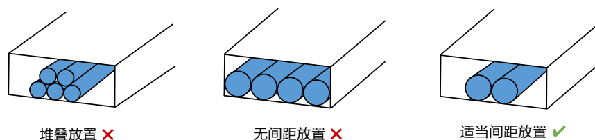
图4-10 线缆铺设后所占据空间
