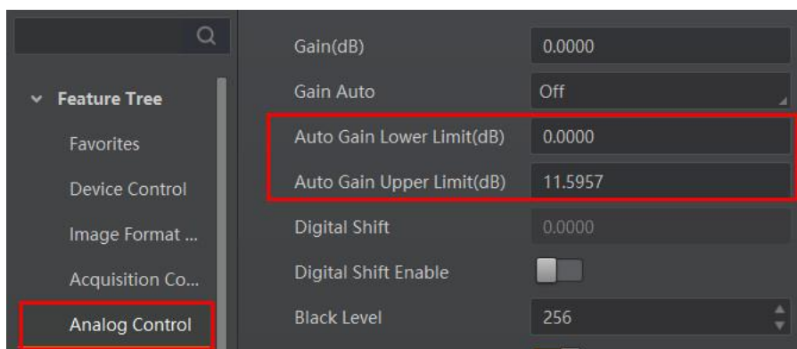
图11-35 模拟增益控制
