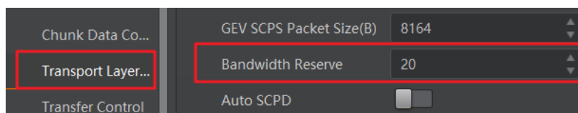
图10-5 预留带宽设置
