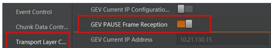
图10-8 Pause 帧接收设置
