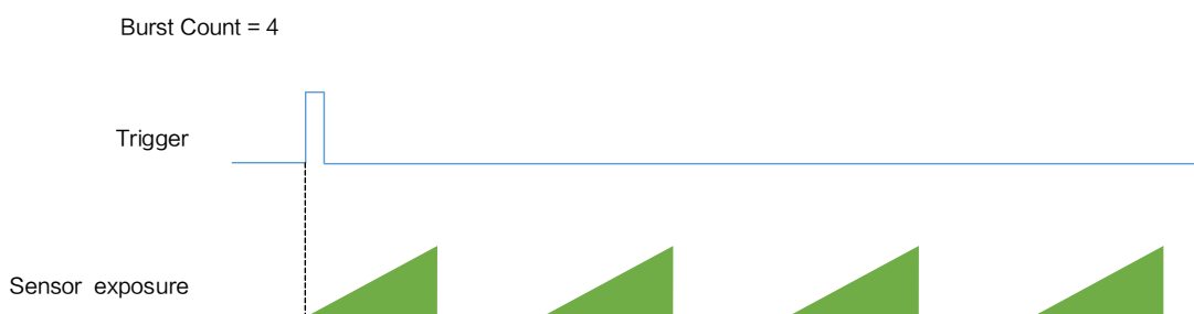
图8-10 触发出图数时序
