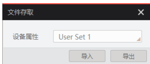
图13-10 导入或导出
