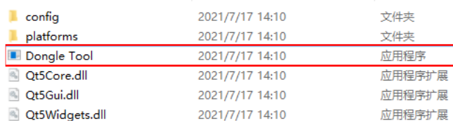
图13-16 Dongle Tool
