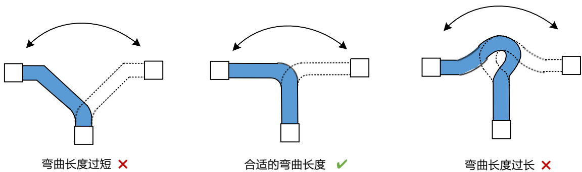
图4-13 预留合适的弯曲长度
