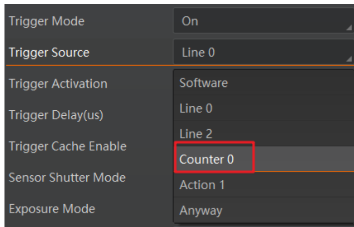
图8-6 计数器触发设置
