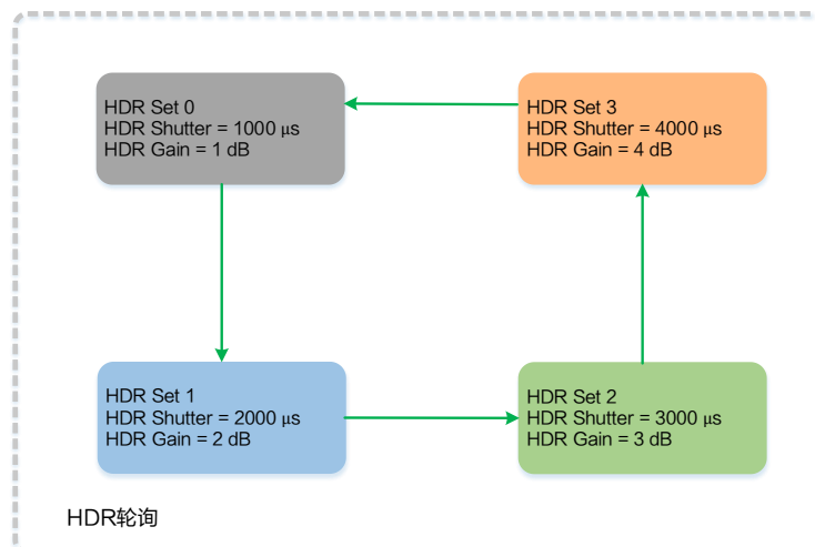
图11-33 HDR 轮询示意图
