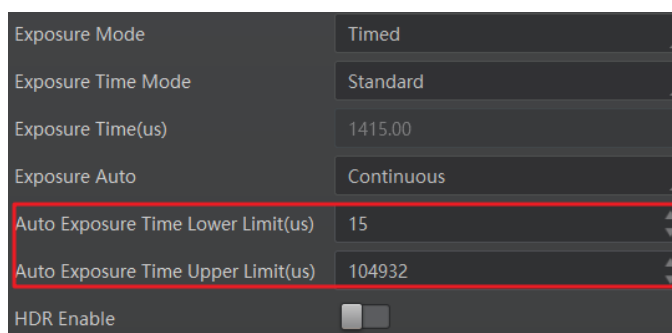
图11-23 曝光时间控制
