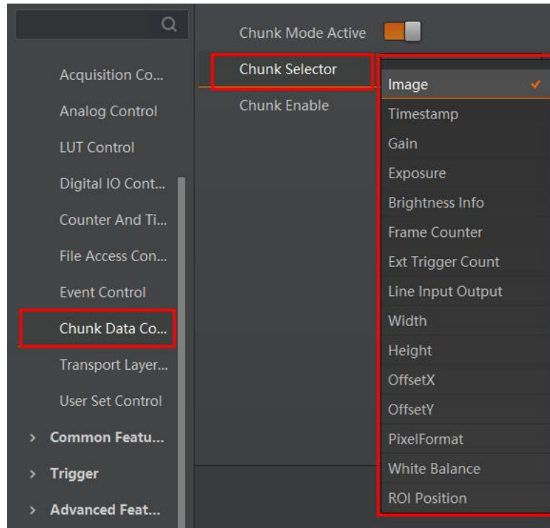
图13-6 选择嵌入的信息
