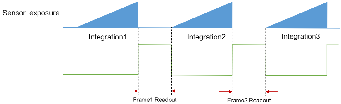
图9-8 内触发模式非交叠曝光
