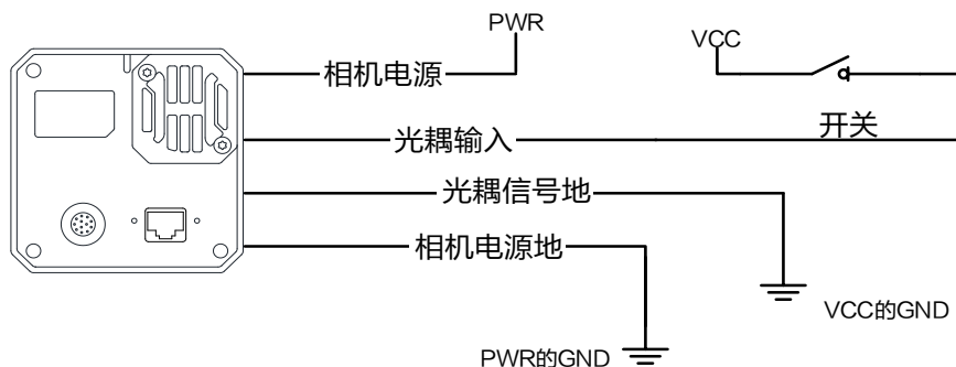
图7-10 Line 0 接开关
