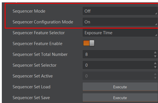
图11-29 Sequencer 配置模式
