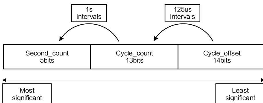
图13-1 Timestamp 数据格式
