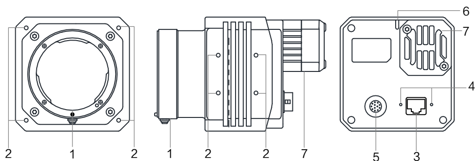
图4-7 F口，带风扇
