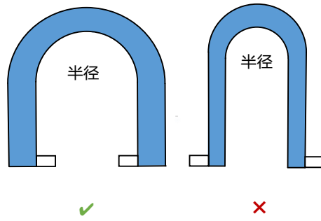
图4-14 足够的弯曲半径
