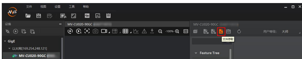
图13-9 文件存取
