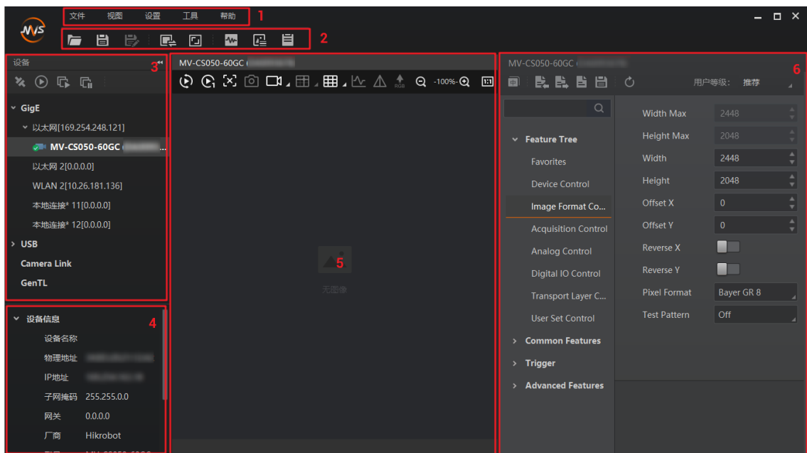
图6-10 软件主界面
