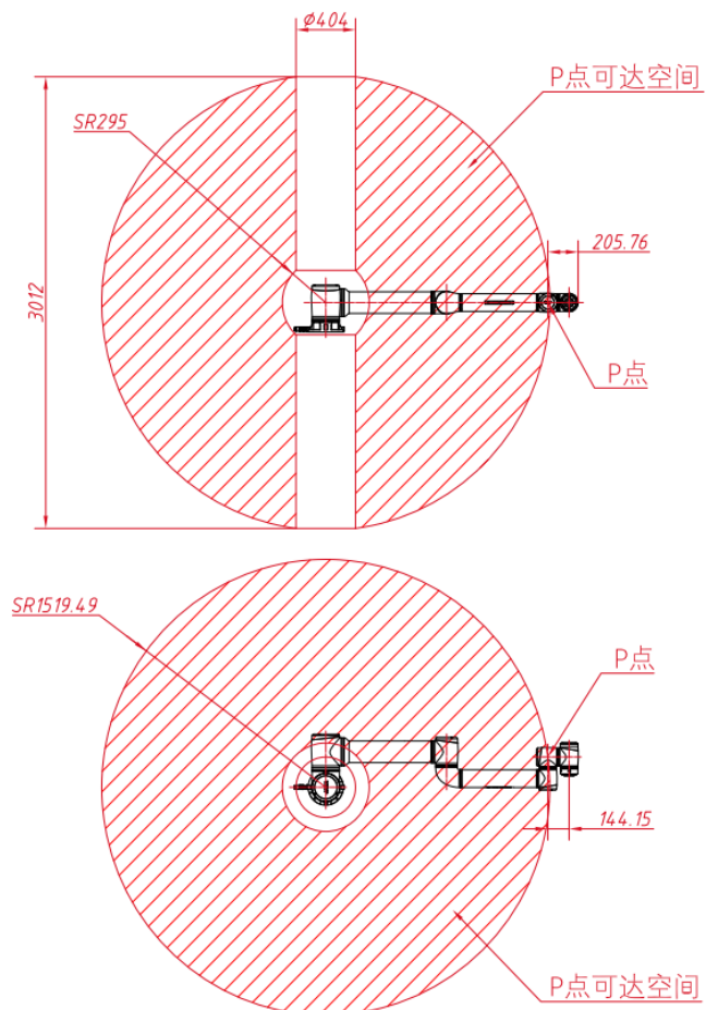
图 3-4 JAKA Zu FT工作空间图
