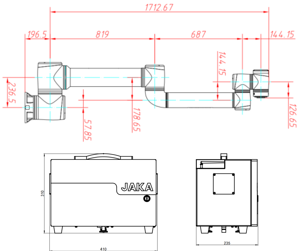
图 3-3 JAKA Zu FT与电控柜外形尺寸图
