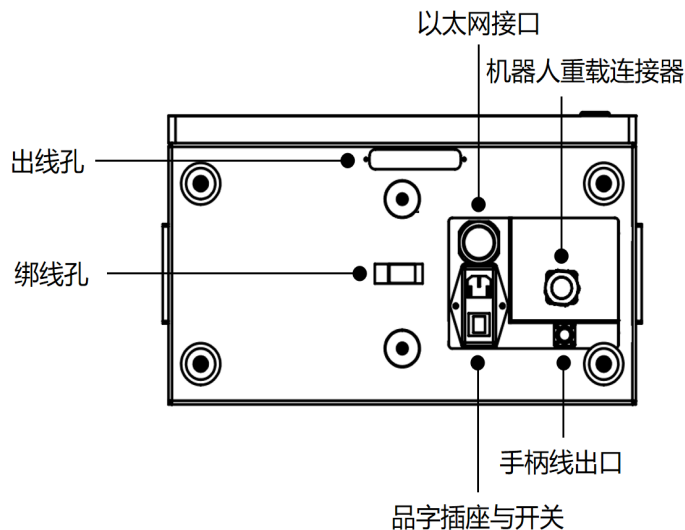
图 4-15 电控柜底面板示意图
