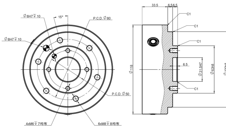
图 3-7 末端法兰安装尺寸图
