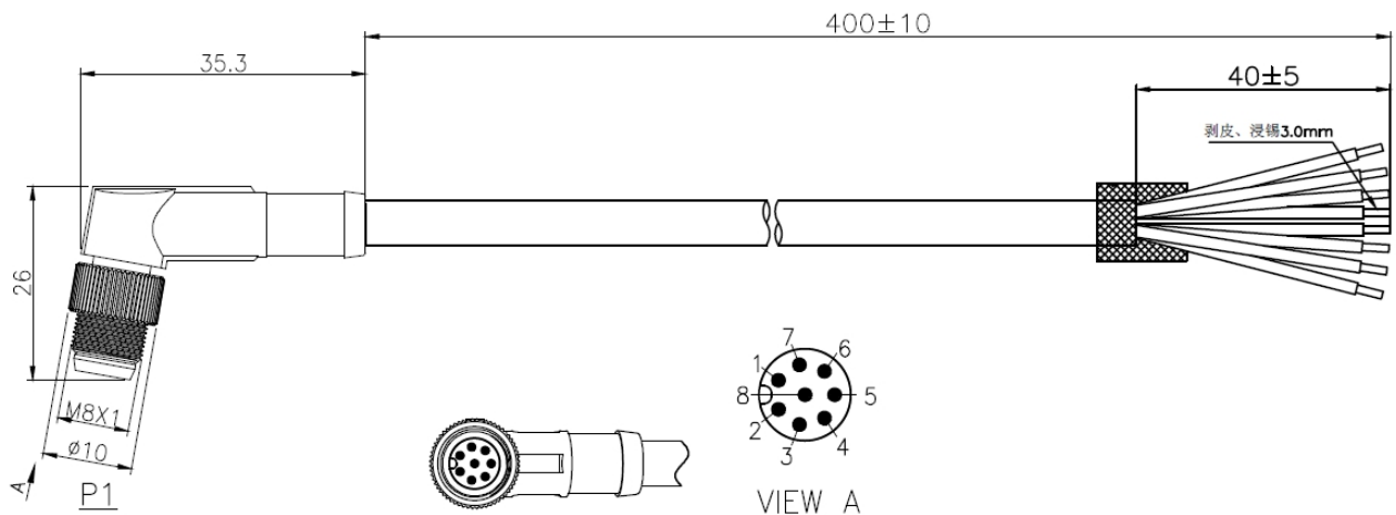
图 4-17 对外连接线
