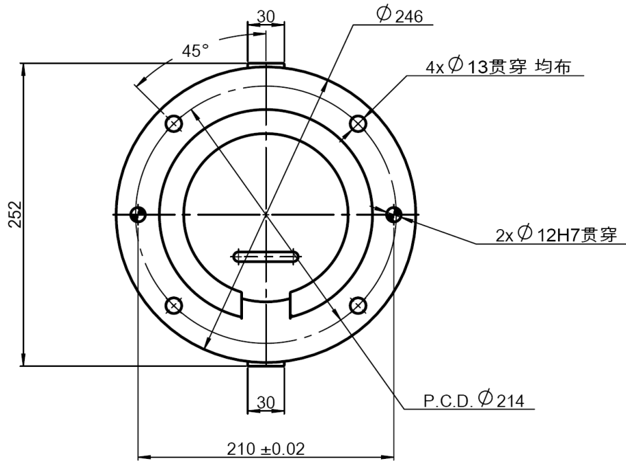
图 3-6 JAKA Zu FT基座安装尺寸图
