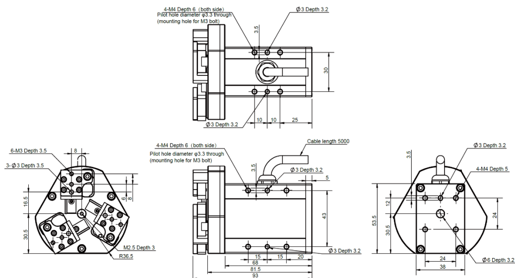
图 1.2 安装尺寸图
