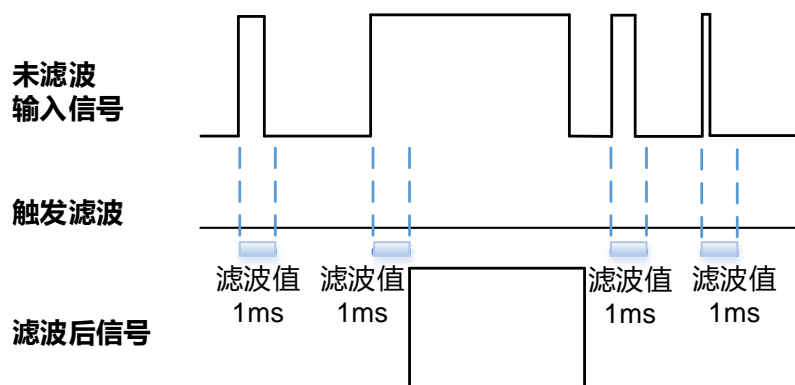
图 8-1 输入信号滤波示意图
