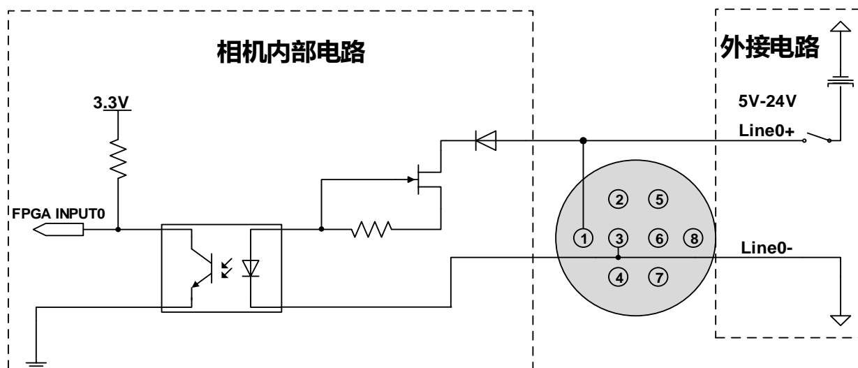
图 7-12 光耦隔离输入电路
