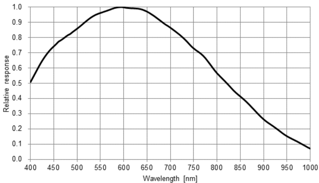
图 4-14 MER2-302-56U3M(-L) SENSOR 响应曲线
