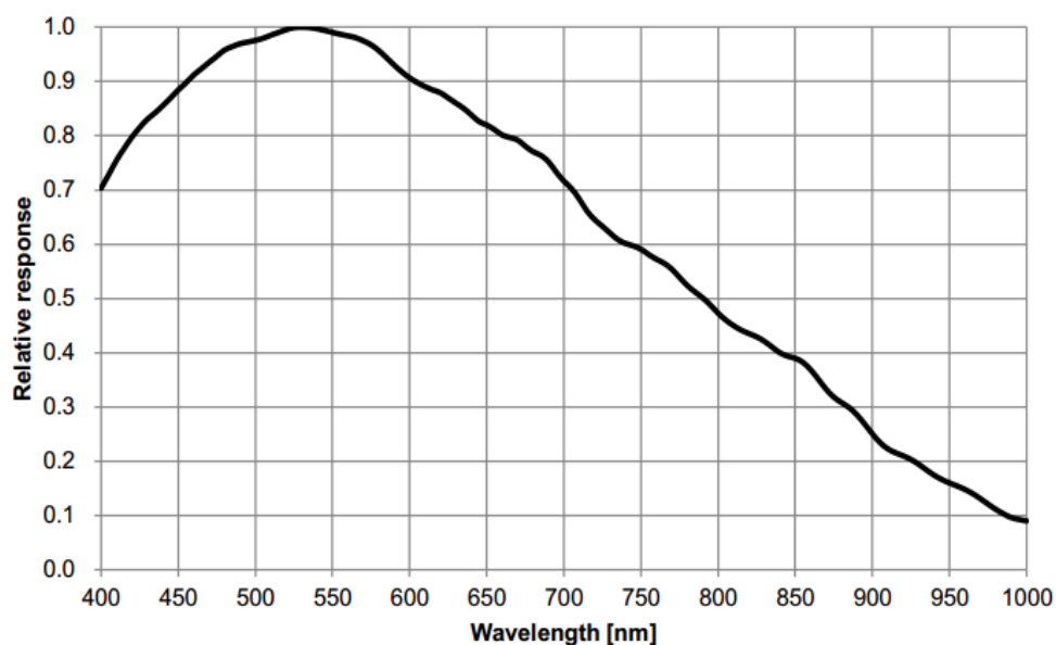
图 4-21 MER2-630-60U3M(-L/-W90) SENSOR 响应曲线
