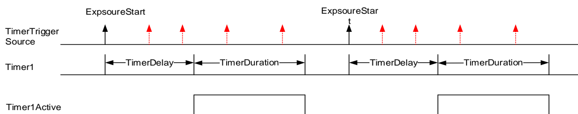
图 8-69 Timer1Active 与曝光开始信号的关系
