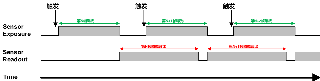
图 8-35 交叠曝光模式下触发采集曝光时序图
