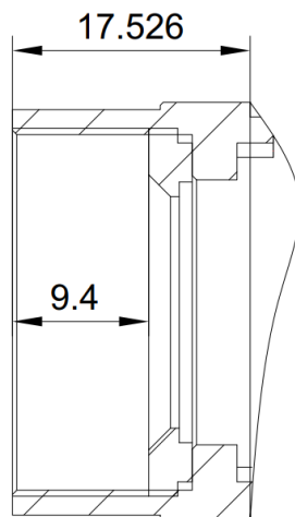
图 5-7 ME2L C 口光学接口
