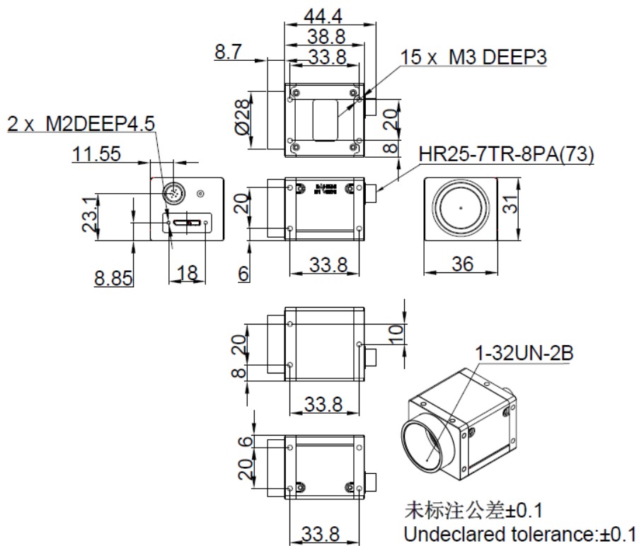
图 5-3 ME2P-U3 机械尺寸图
