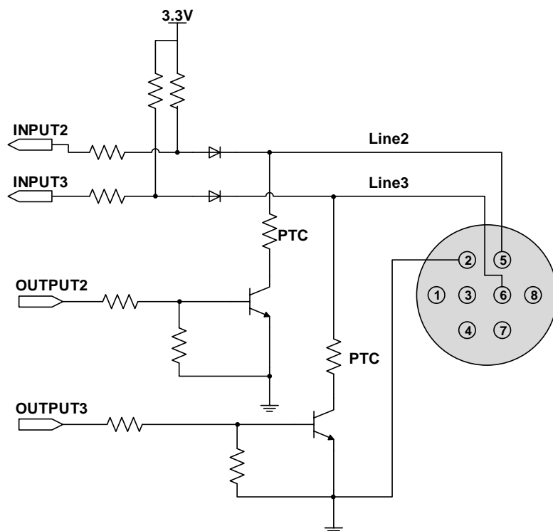
图 7-7 GPIO 2/3 (双向) 电路
