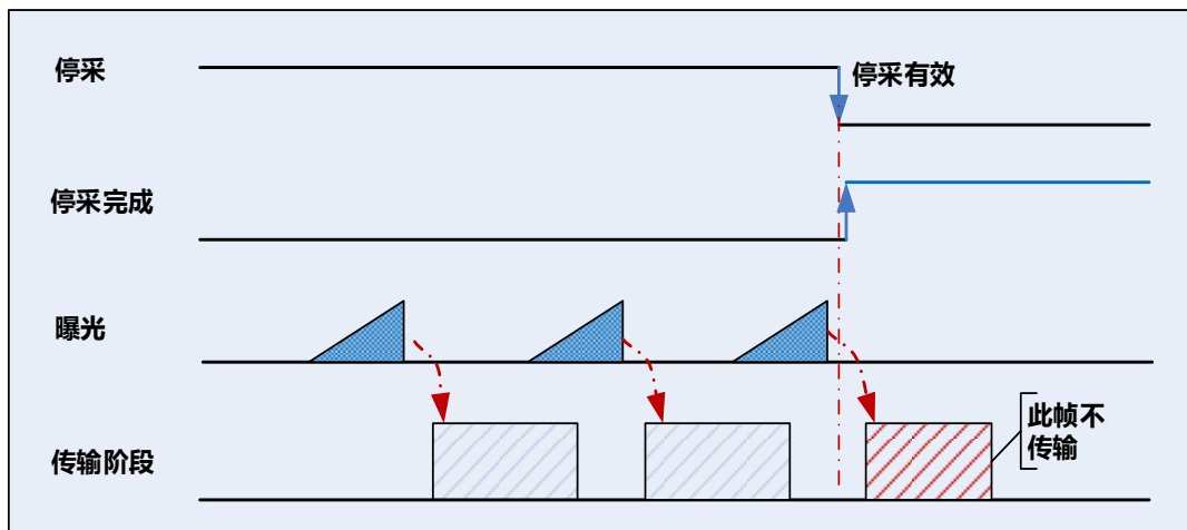
图 8-18 传输等待时停采时序图
