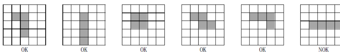
图 4-34 ME2P-2622-15U3M NIR 连续坏点分布情况示意图
