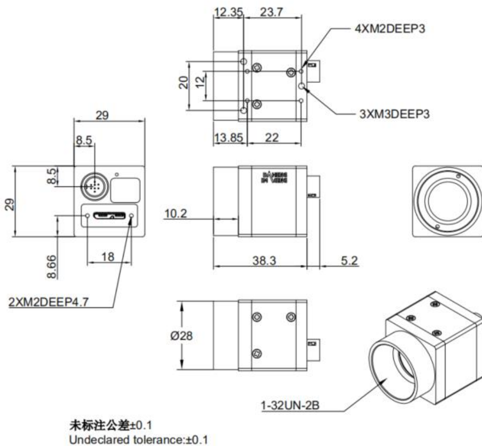
图 5-4 ME2L-U3 机械尺寸图
