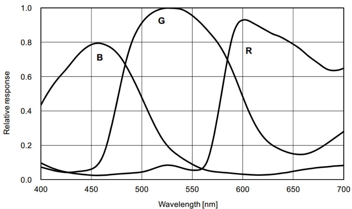
图 4-24 MER2-2000-19U3C(-L/-W90) SENSOR 响应曲线
