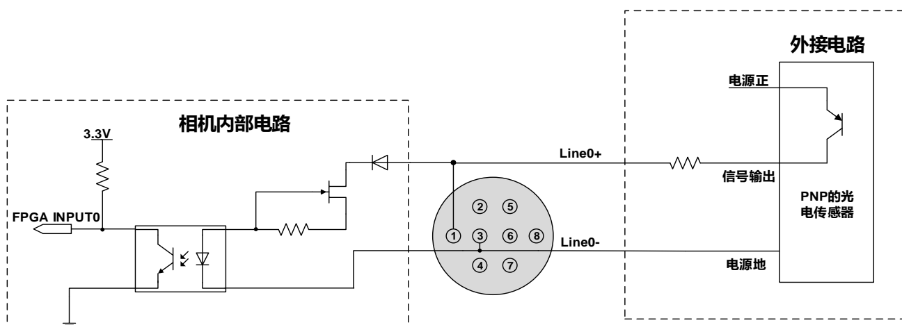
图 7-14 PNP 型光电传感器连接到光耦隔离输入电路
