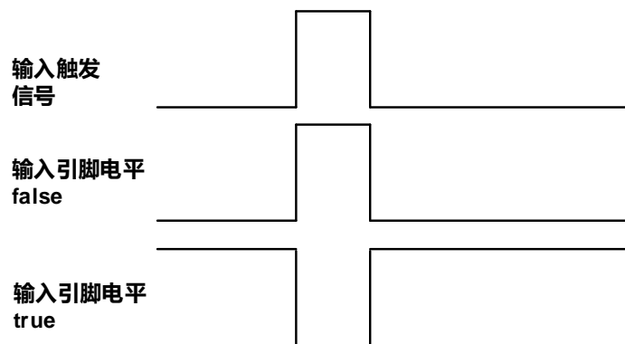
图 8-12 设置输入引脚反向
