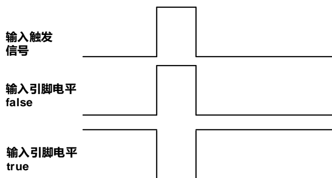
图 8-3 设置输入引脚反向
