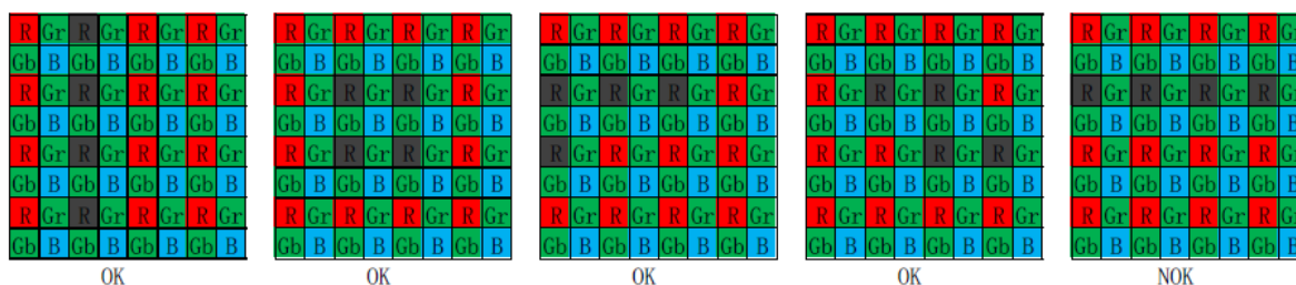
图 4-31 ME2P-2622-15U3C 连续坏点为相同颜色分量分布情况示意图
