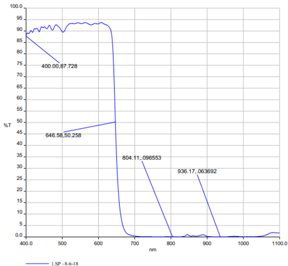
图 6-1 水星二代彩色相机滤色片透过率曲线
