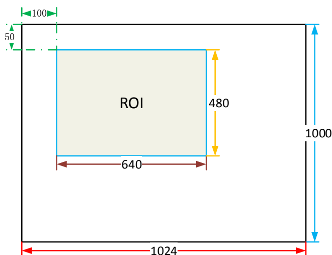
图 8-42 自动白平衡 ROI 与当前图像关系示意图
