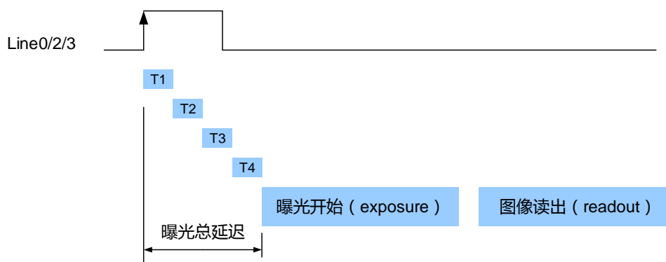
图 8-24 曝光延迟
