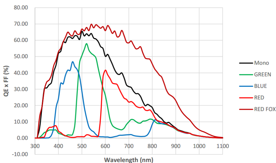
图 4-35 ME2P-2621-15U3M NIR \ ME2P-2622-15U3M NIR SENSOR 响应曲线
