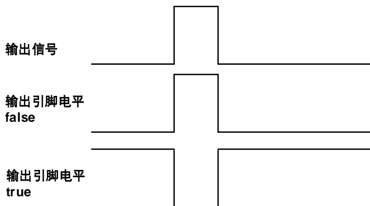
图 8-14 设置输出引脚反向
