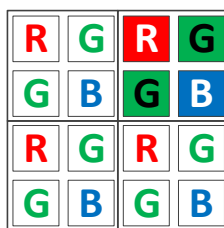
图 8-52 彩色相机水平垂直 Binning 系数 2x2
