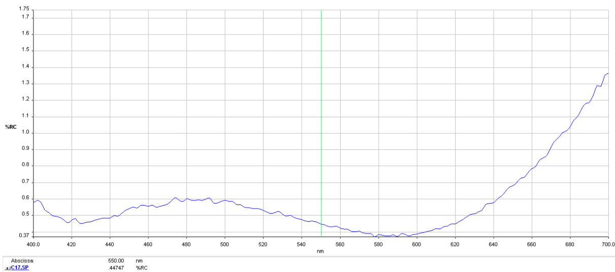
图 6-2 水星二代黑白相机透光片反射率曲线
