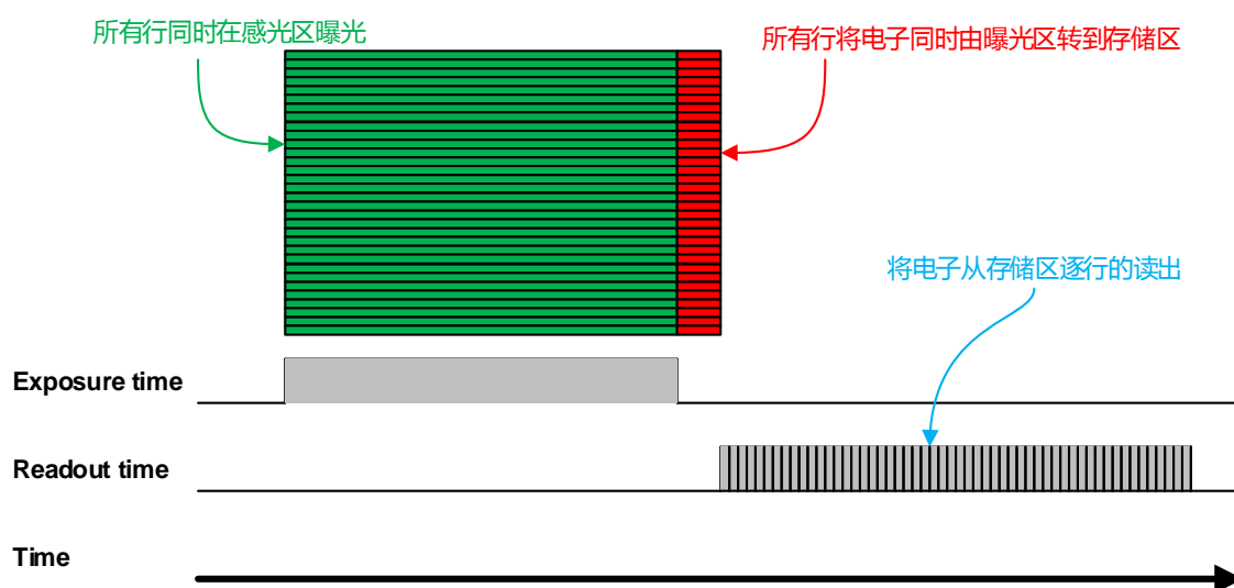
图 8-29 全局曝光模式
