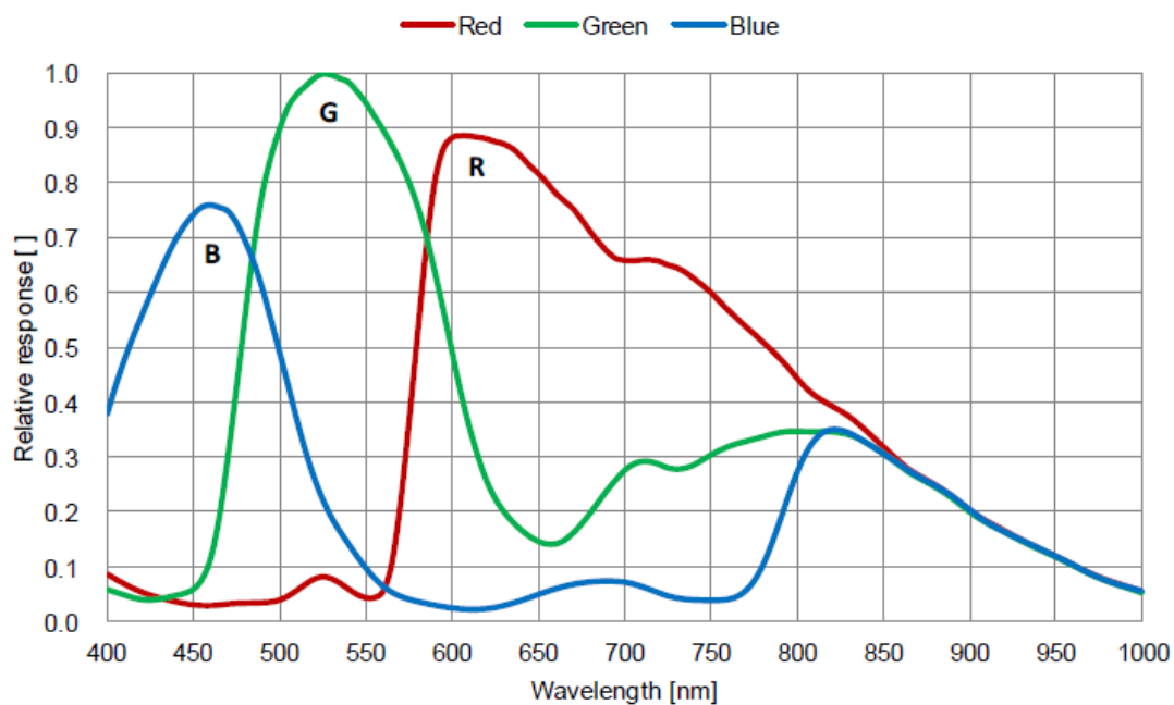
图 4-7 MER2-230-168U3C(-L) SENSOR 响应曲线
