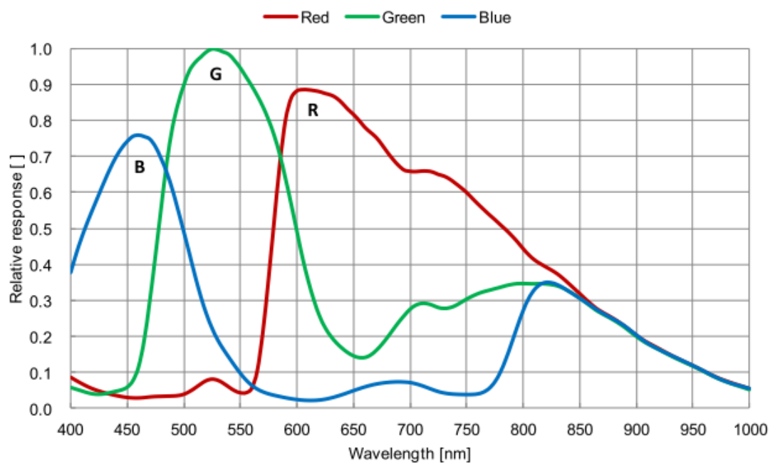
图 4-9 MER2-231-41U3C(-L) SENSOR 响应曲线
