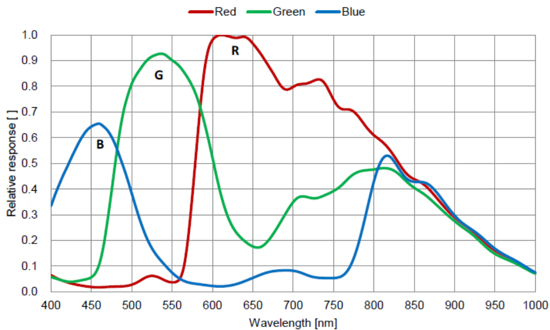
图 4-11 MER2-301-125U3C(-L) SENSOR 响应曲线
