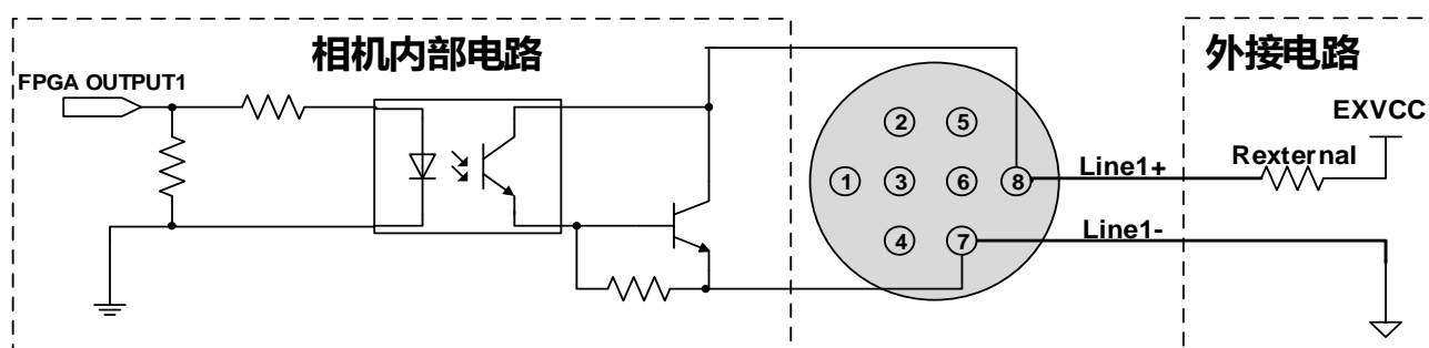
图 7-5 光耦隔离输出电路
