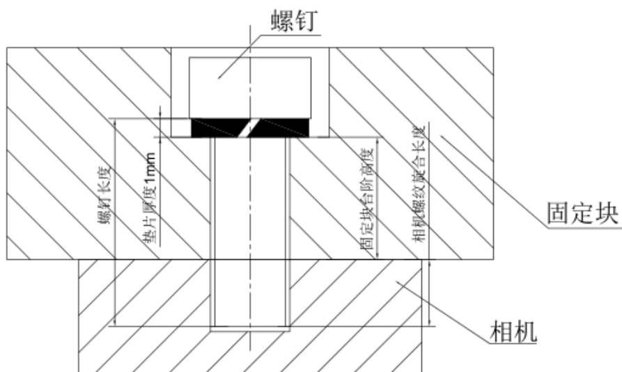
图 5-8 螺钉规格、固定块台阶厚度、弹垫厚度关系图
