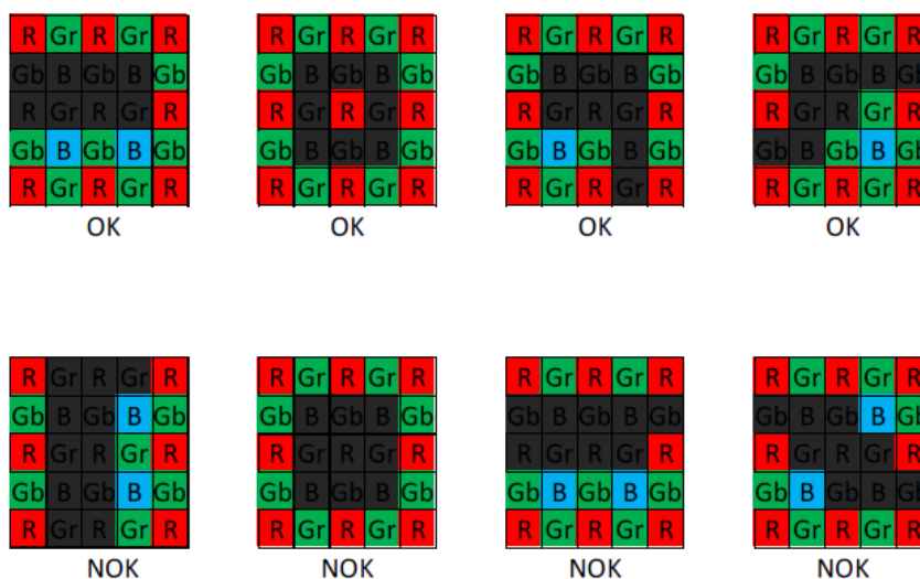
图 4-32 ME2P-2622-15U3C 连续坏点为不同颜色分量分布情况示意图
