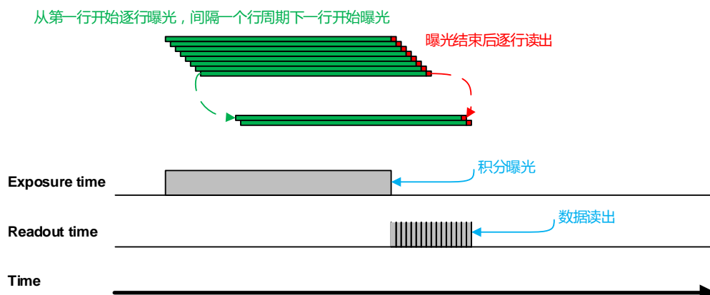
图 8-30 逐行曝光模式
