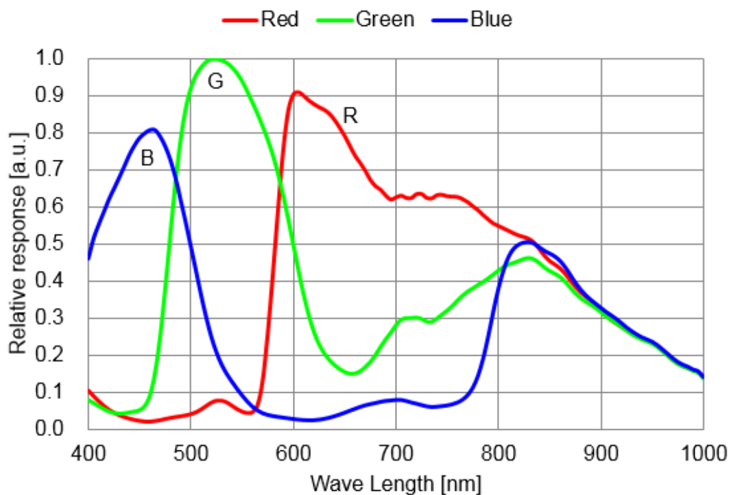
图 4-38 ME2L-505-36U3C(-L) SENSOR 响应曲线
