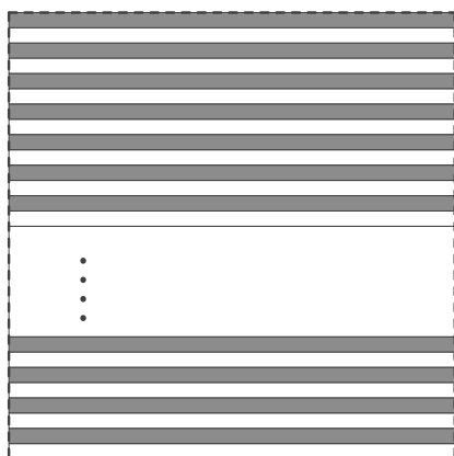
图 8-54 黑白相机垂直像素抽样原理
