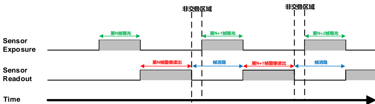
图 8-32 非交叠曝光模式下曝光时序图
