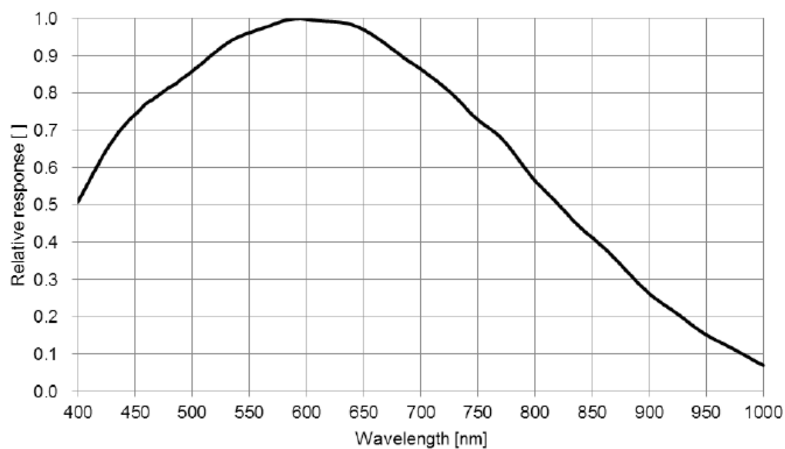
图 4-12 MER2-301-125U3M(-L) SENSOR 响应曲线
