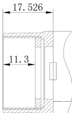
图 5-6 ME2P/MER2 C 口光学接口
