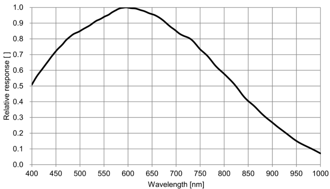
图 4-29 ME2P-1231-32U3M SENSOR 响应曲线
