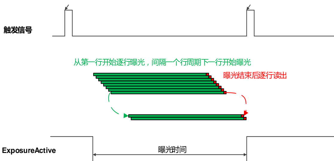
图 8-6 逐行曝光 ExposureActive 信号示意图
