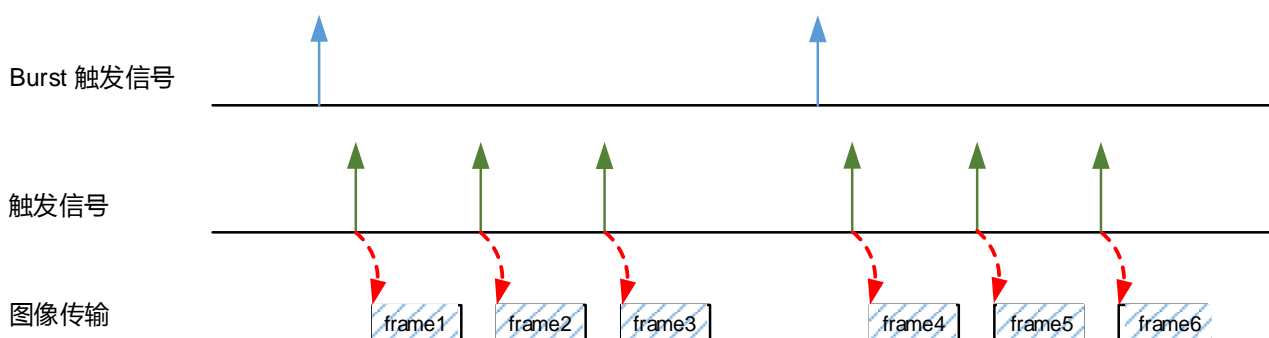
图 8-21 触发模式同时打开触发时序图
