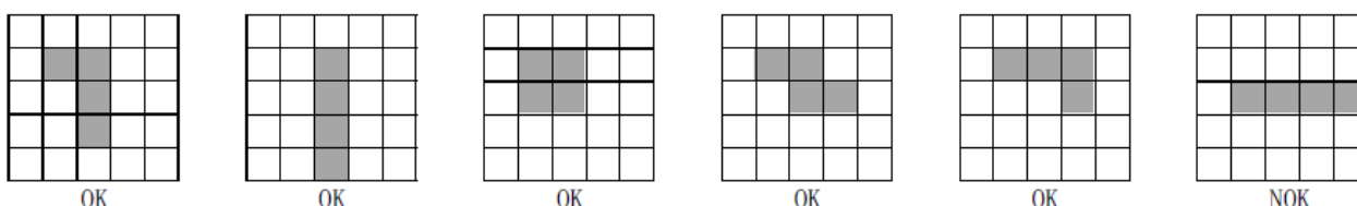
图 4-30 ME2P-2622-15U3M 连续坏点分布情况示意图
