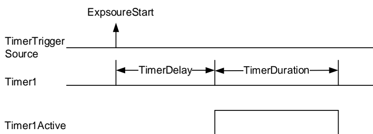
图 8-68 Timer1Active 示意图
