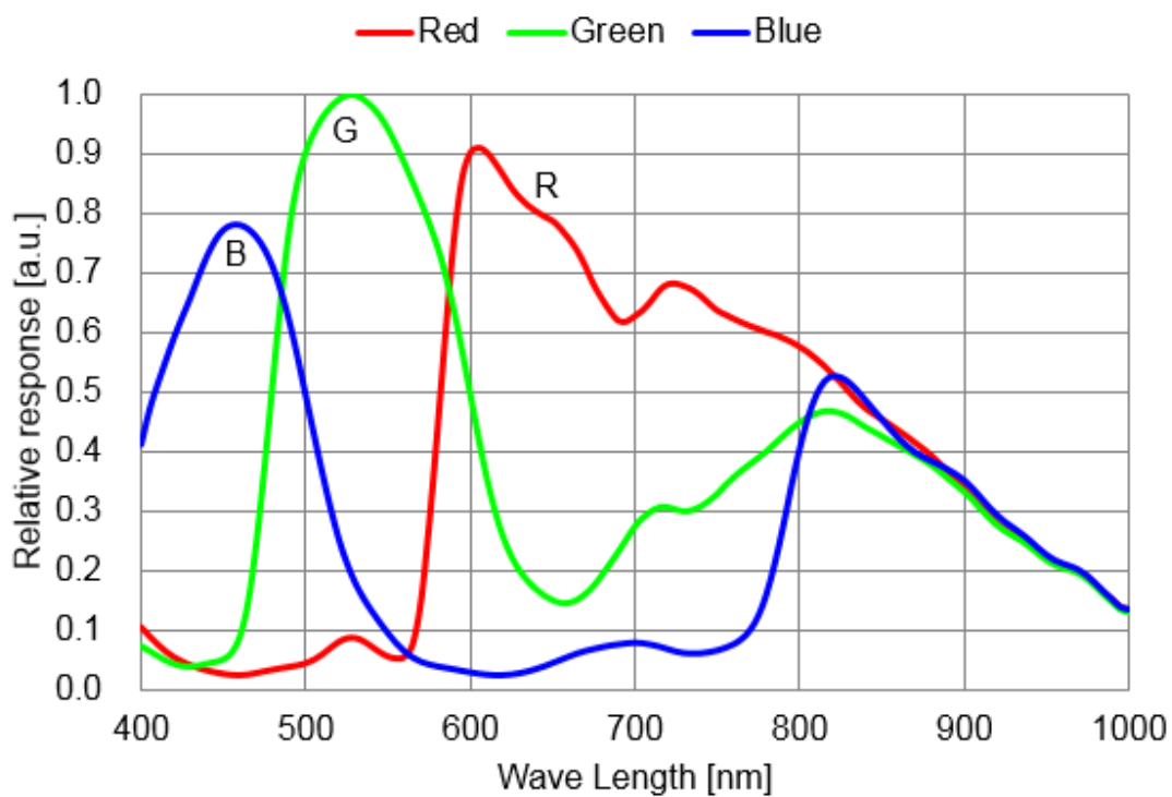
图 4-40 ME2L-830-22U3C(-L) SENSOR 响应曲线
