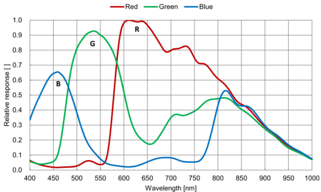
图 4-15 MER2-502-79U3C(-L) SENSOR 响应曲线
