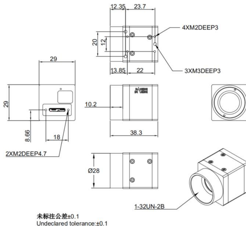
图 5-5 ME2L-U3-L 机械尺寸图
