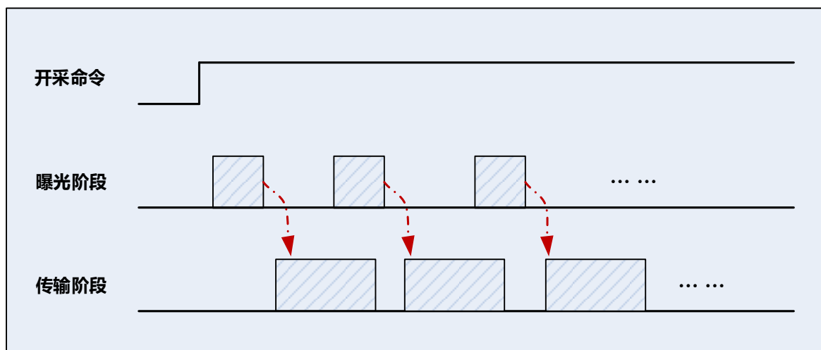
图 8-15 连续采集时序图
