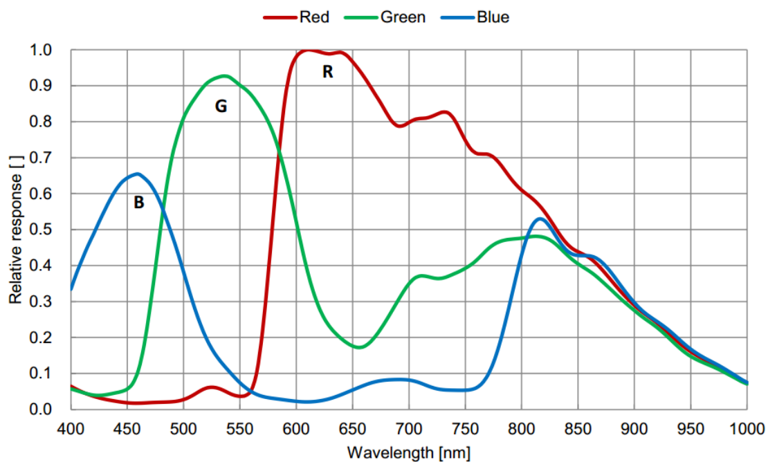
图 4-17 MER2-503-36U3C(-L) SENSOR 响应曲线
