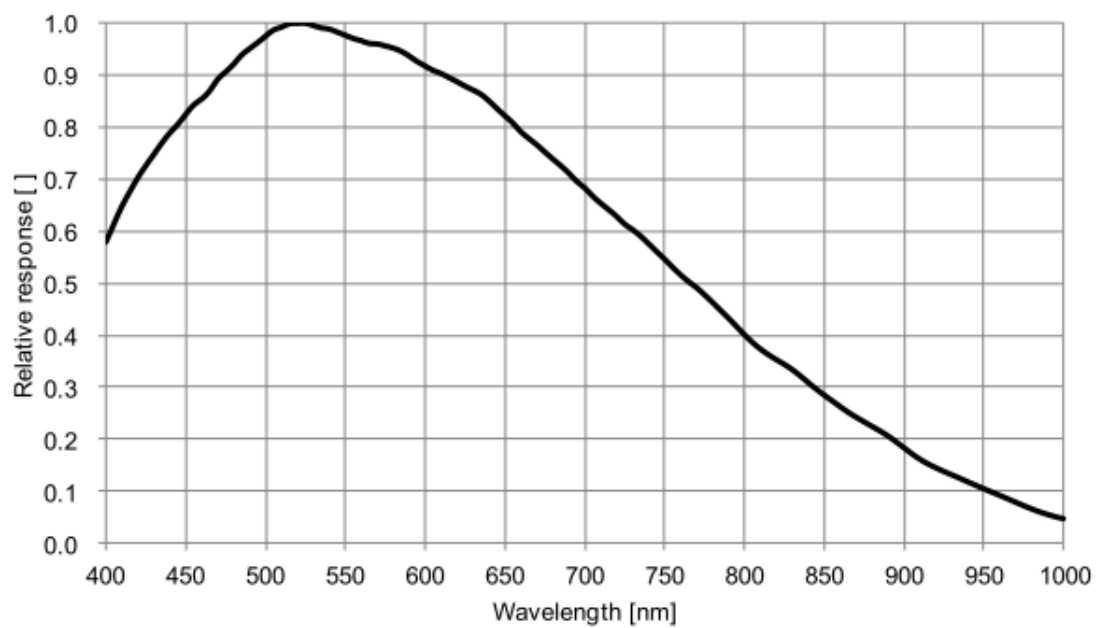
图 4-10 MER2-231-41U3M(-L) SENSOR 响应曲线
