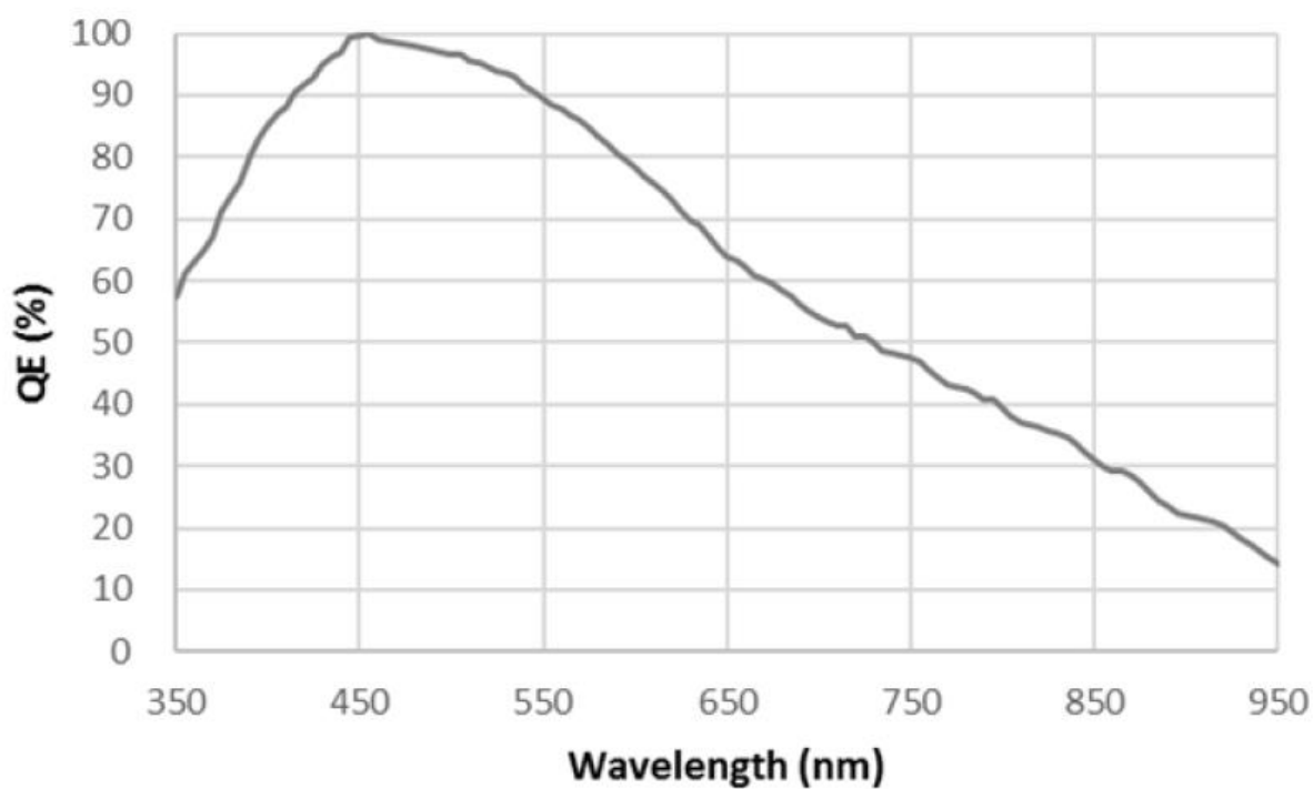
图 4-4 MER2-135-208U3M(-L) SENSOR 响应曲线
