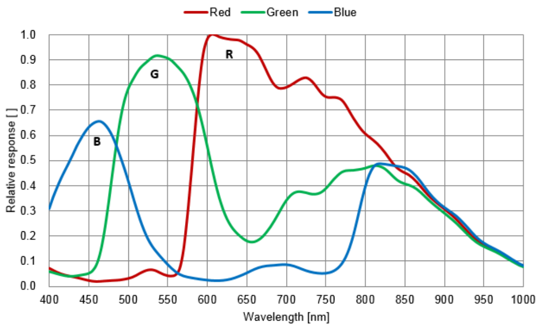
图 4-36 ME2L-161-61U3C(-L) SENSOR 响应曲线
