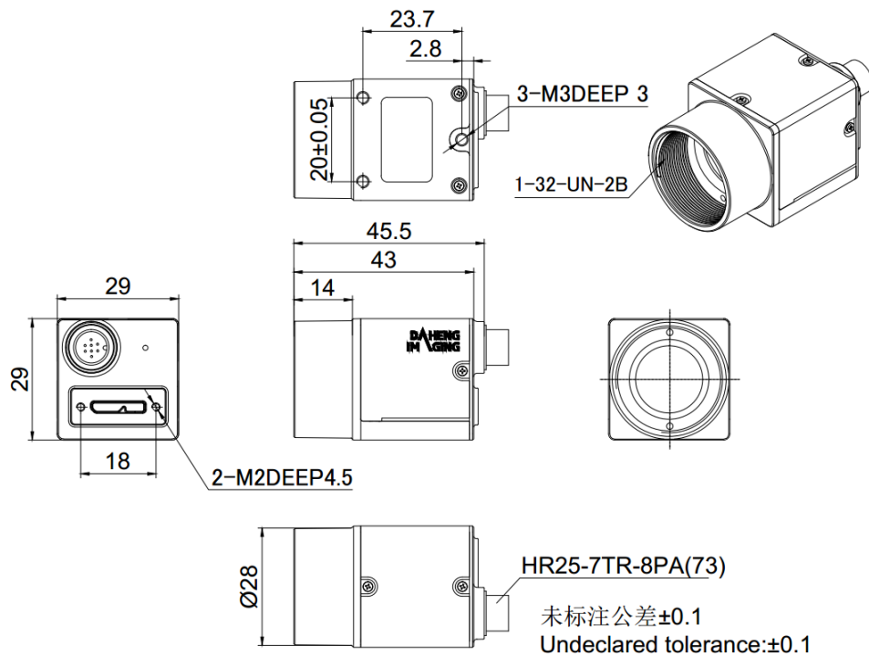
图 5-1 MER2-U3 机械尺寸图
