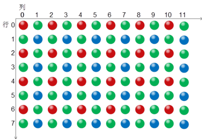
图 8-38 BayerRG8 的像素排列示意图
