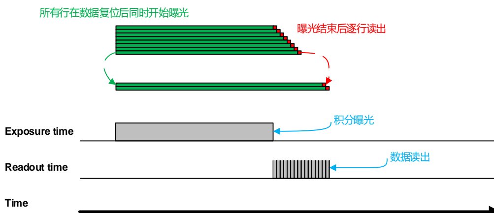
图 8-31 全局复位释放模式
