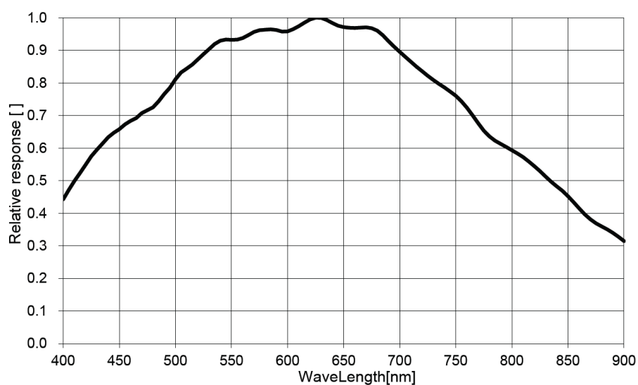
图 4-19 MER2-503-36U3M POL SENSOR 响应曲线
