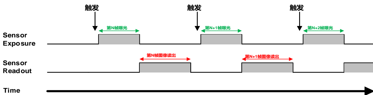
图 8-33 非交叠曝光模式下触发采集曝光时序图
