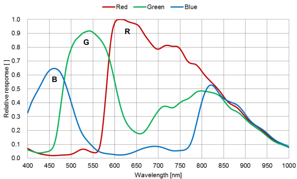
图 4-26 ME2P-1230-23U3C SENSOR 响应曲线
