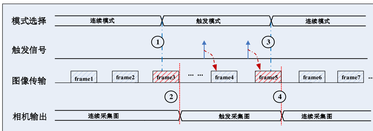
图 8-22 传输时切换触发模式
