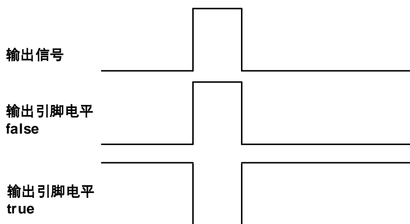
图 8-9 设置输出引脚反向
