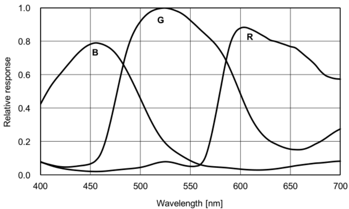
图 4-22 MER2-1220-32U3C(-L/-W90) SENSOR 响应曲线
