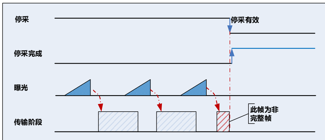
图 8-17 传输过程中停采时序图
