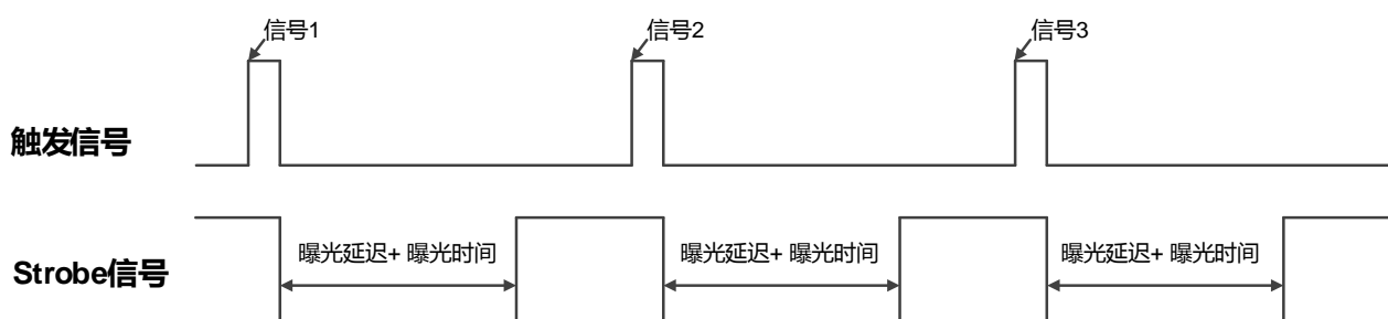
图 8-13 Strobe 信号示意图
