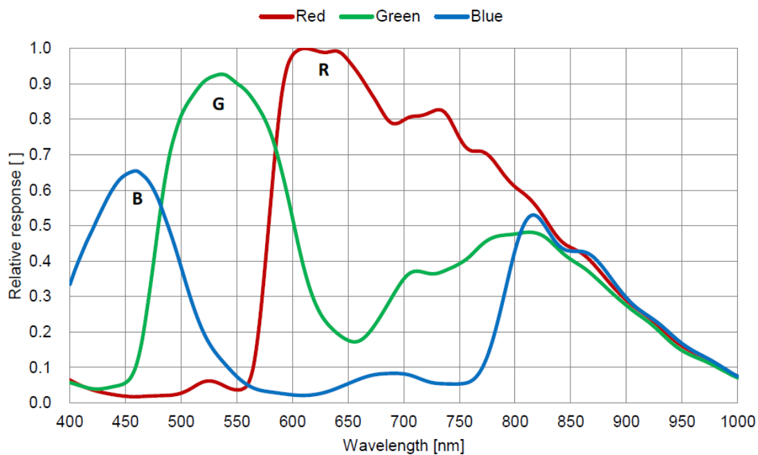
图 4-13 MER2-302-56U3C(-L) SENSOR 响应曲线
