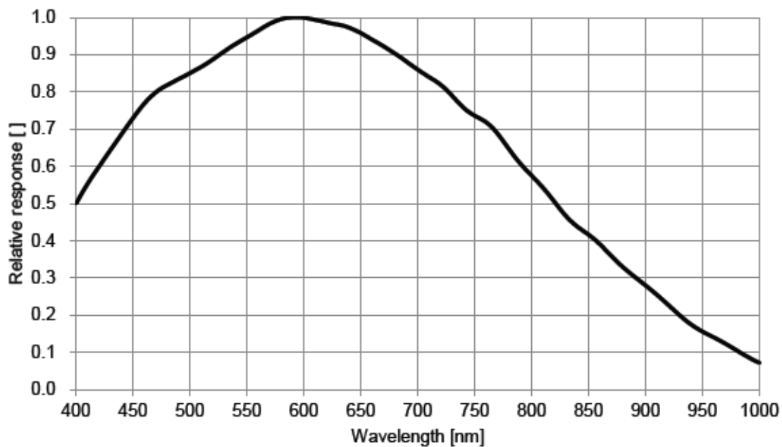
图 4-6 MER2-160-227U3M(-L) SENSOR 响应曲线
