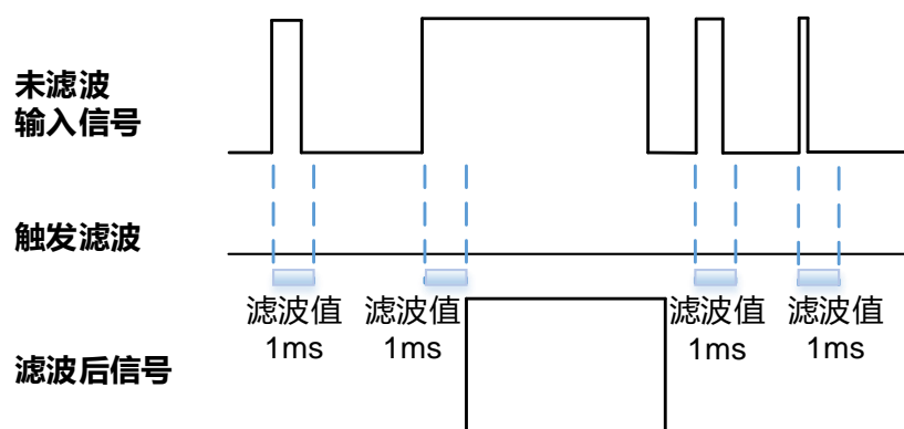
图 8-10 输入信号滤波示意图
