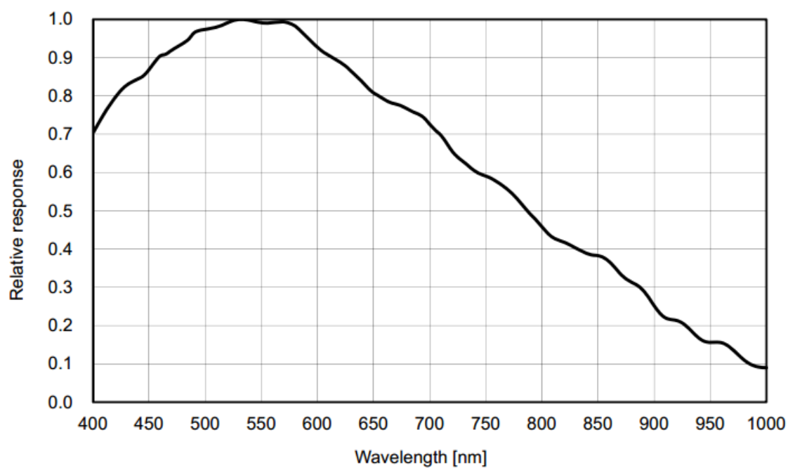
图 4-25 MER2-2000-19U3M(-L/-W90) SENSOR 响应曲线
