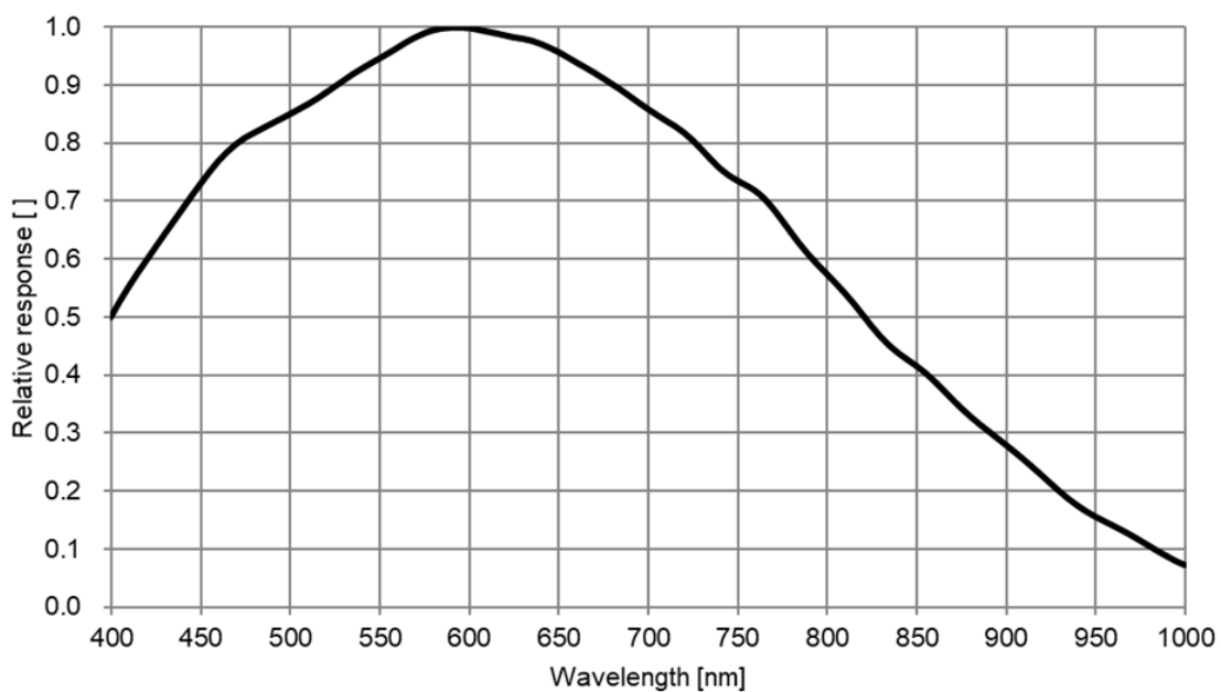
图 4-37 ME2L-161-61U3M(-L) SENSOR 响应曲线
