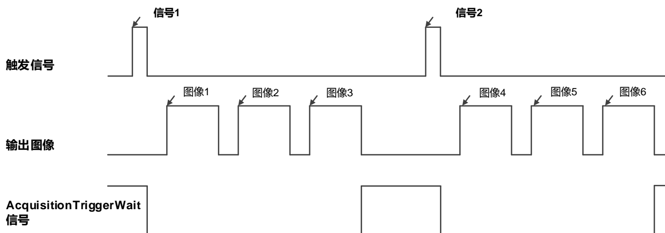
图 8-8 AcquisitionTriggerWait 信号示意图
