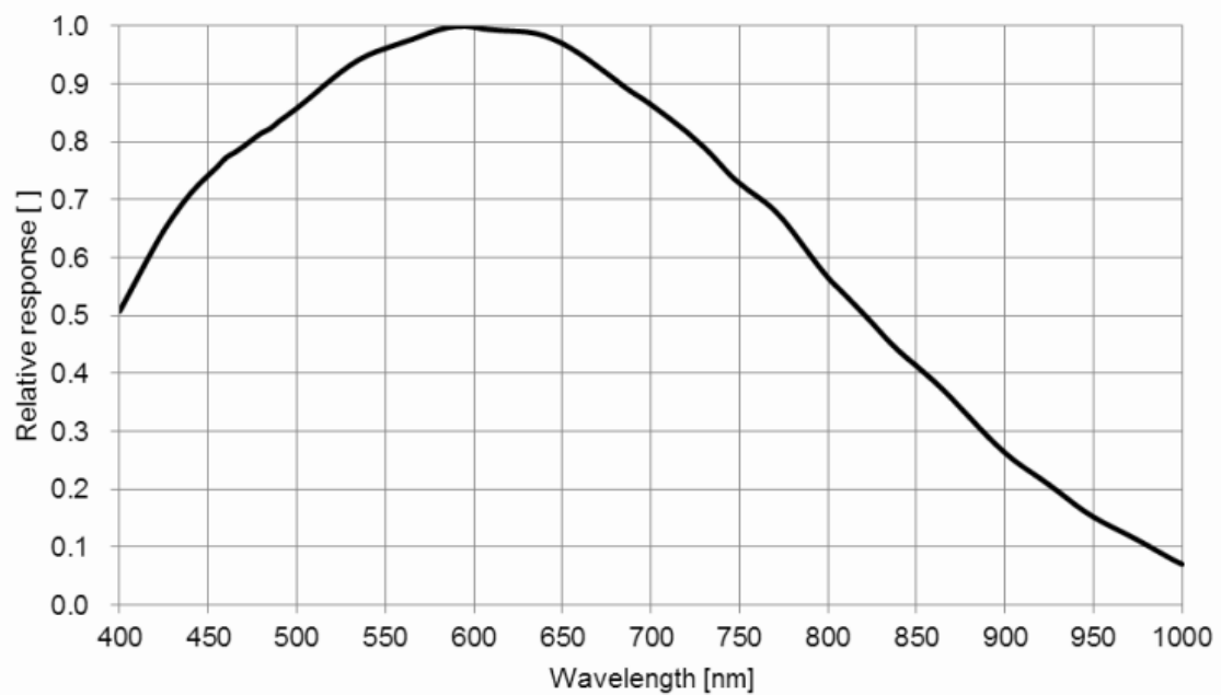
图 4-16 MER2-502-79U3M(-L) SENSOR 响应曲线
