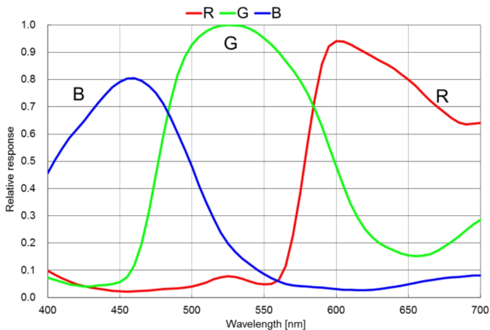
图 4-20 MER2-630-60U3C(-L/-W90) SENSOR 响应曲线
