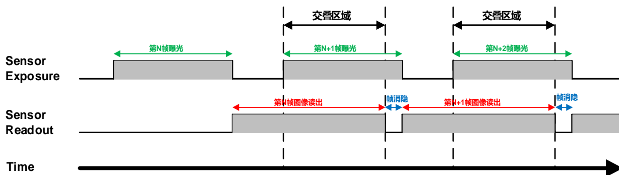
图 8-34 交叠曝光模式下曝光时序图
