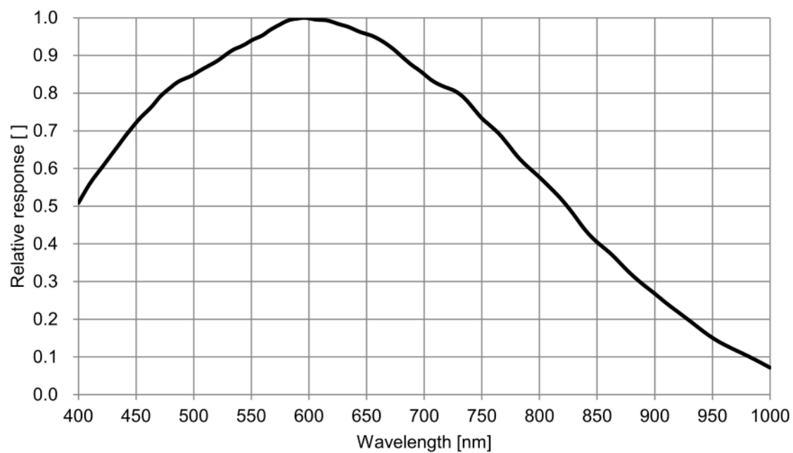
图 4-27 ME2P-1230-23U3M SENSOR 响应曲线
