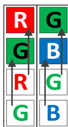
图 8-51 彩色相机垂直 Binning 系数为 2
