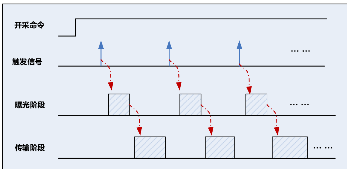
图 8-16 触发采集时序图
