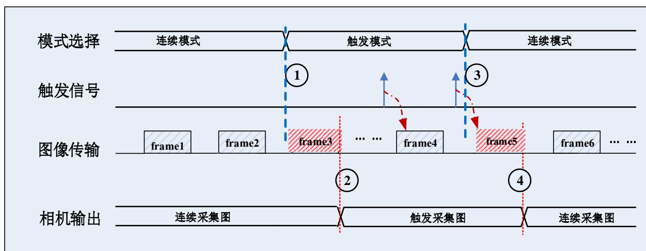
图 8-23 传输等待时切换触发模式
