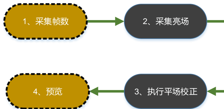
图 8-79 平场校正系数求取流程图
