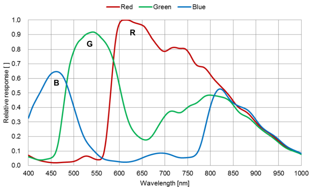
图 4-28 ME2P-1231-32U3C SENSOR 响应曲线
