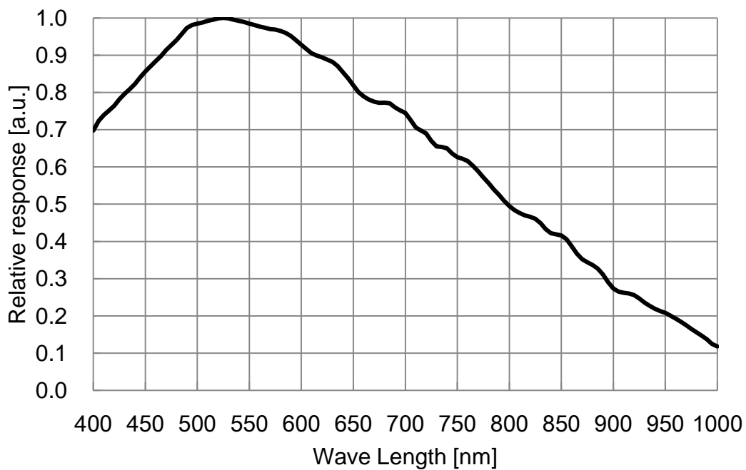
图 4-41 ME2L-830-22U3M(-L) SENSOR 响应曲线
