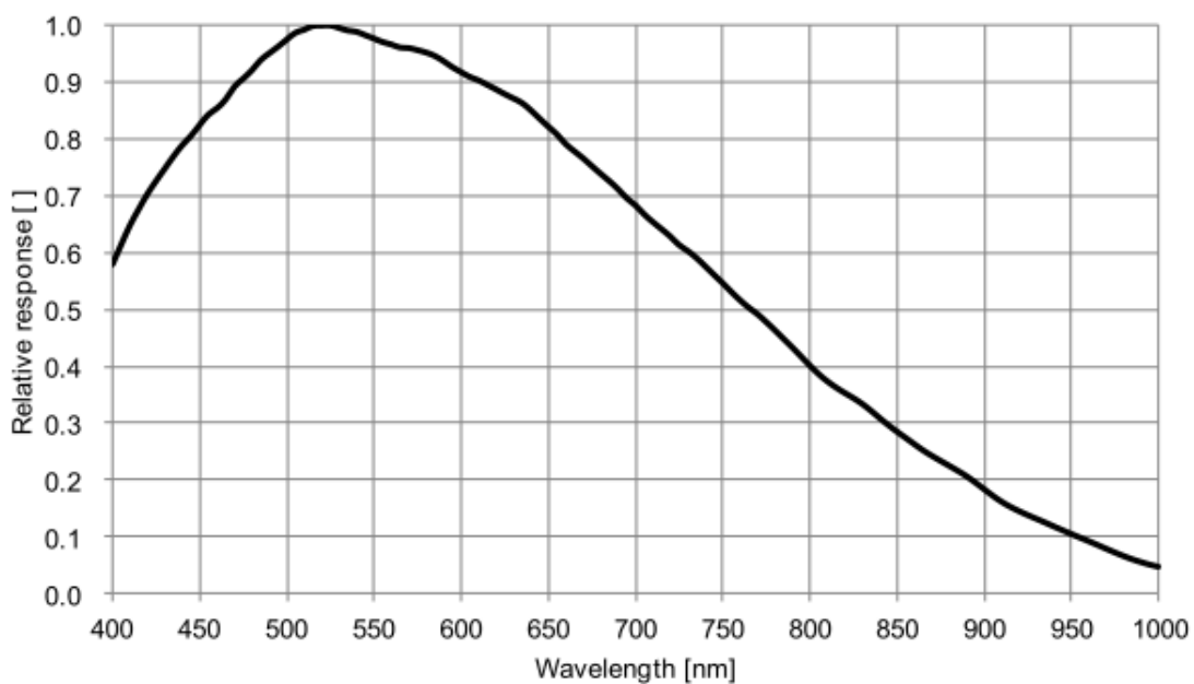
图 4-8 MER2-230-168U3M(-L) SENSOR 响应曲线
