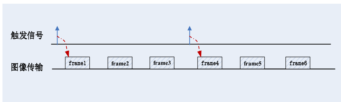
图 8-20 帧高速连拍开始触发时序图
