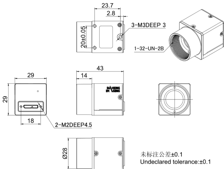
图 5-2 MER2-U3-L 机械尺寸图
