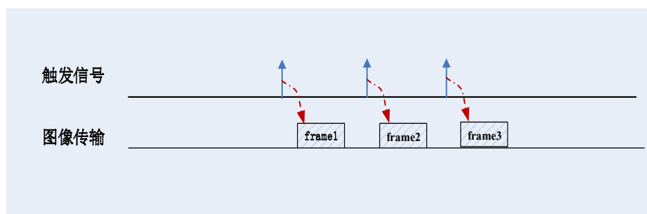
图 8-19 帧开始触发时序图
