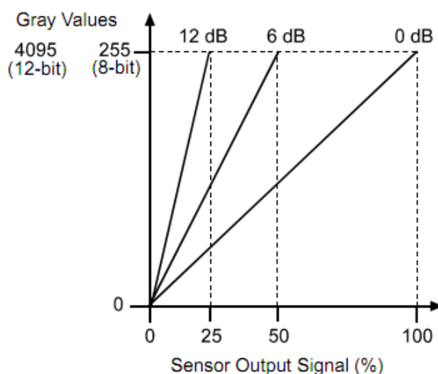
图 8-36 相机响应曲线
