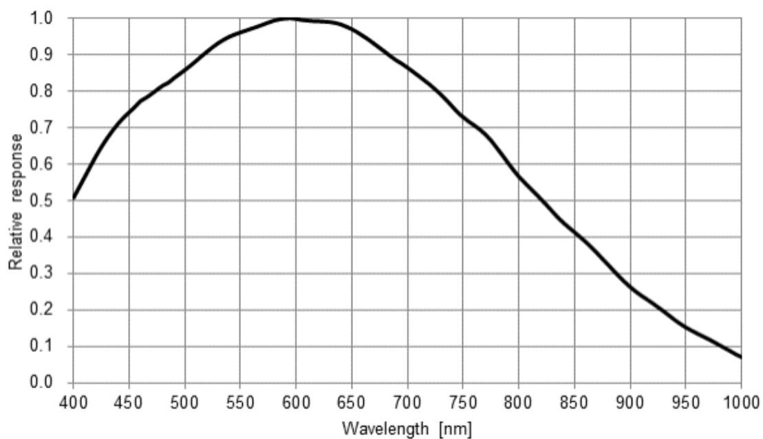
图 4-18 MER2-503-36U3M(-L) SENSOR 响应曲线
