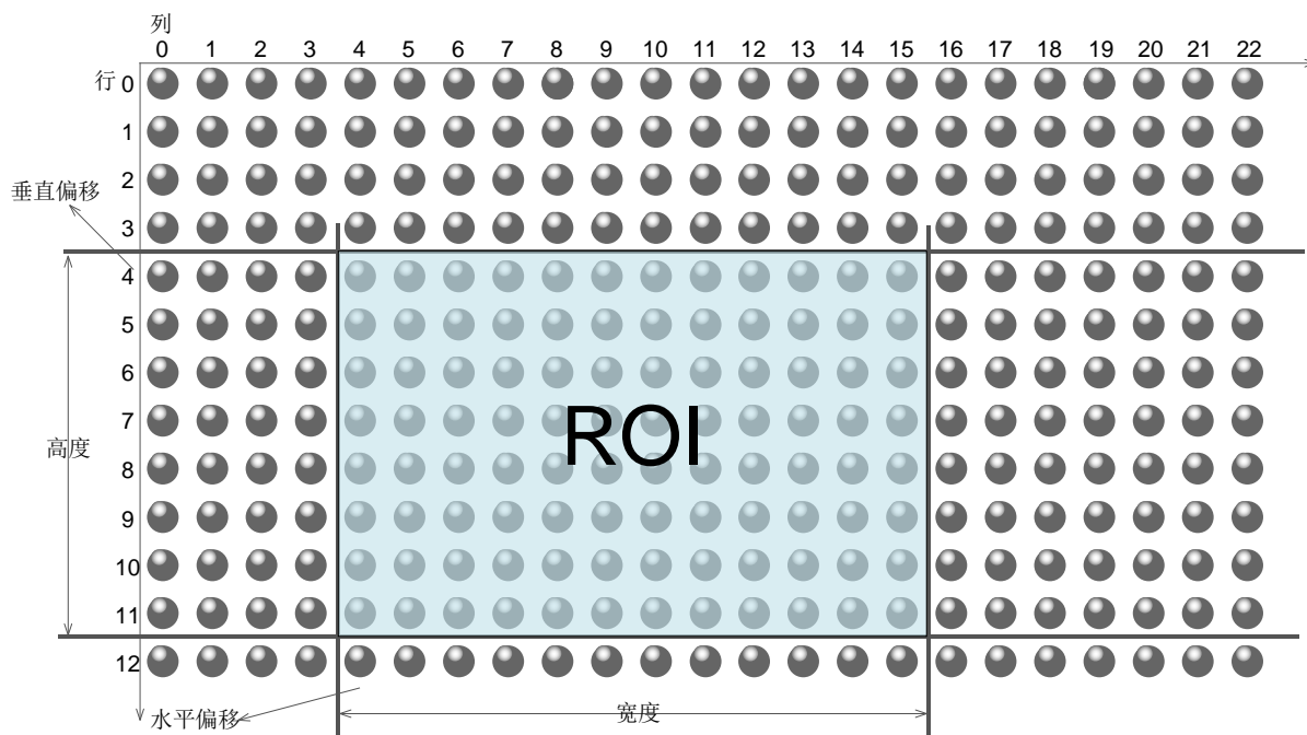
图 8-39 ROI 示意图
