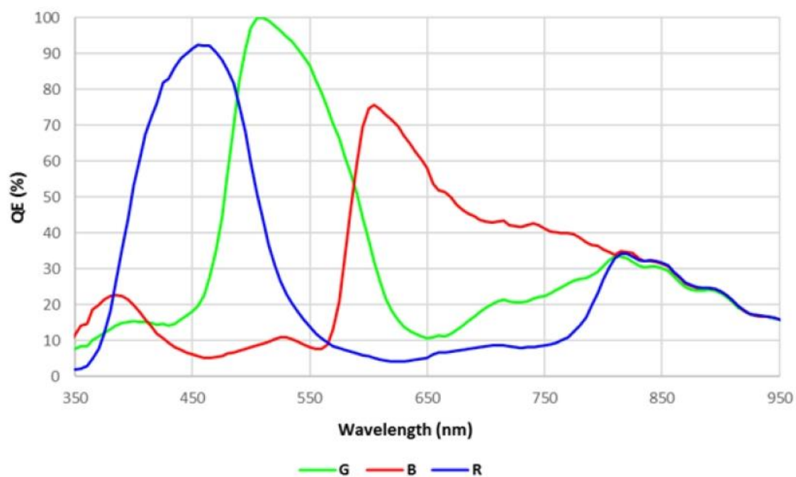
图 4-3 MER2-135-208U3C(-L) SENSOR 响应曲线
