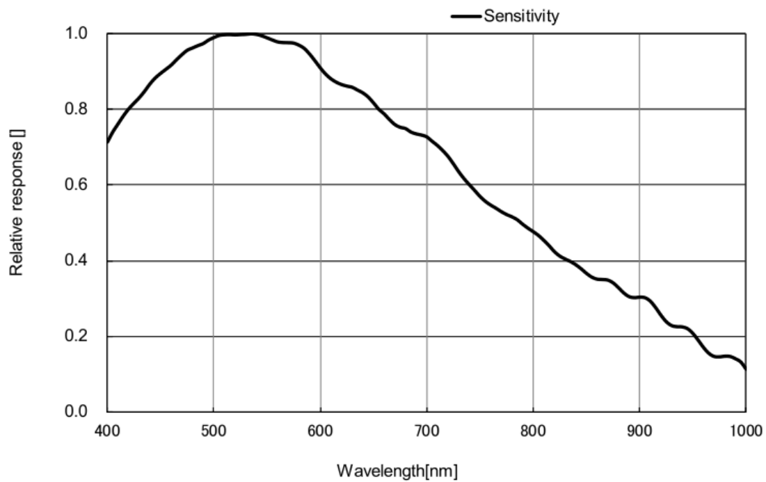
图 4-23 MER2-1220-32U3M(-L/-W90) SENSOR 响应曲线
