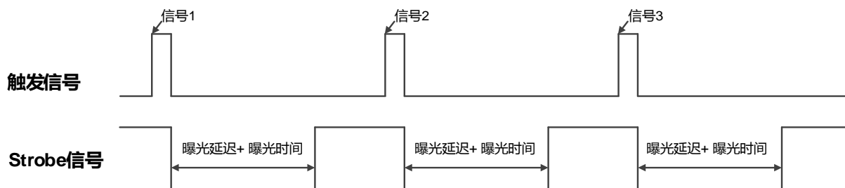
图 8-4 Strobe 信号示意图
