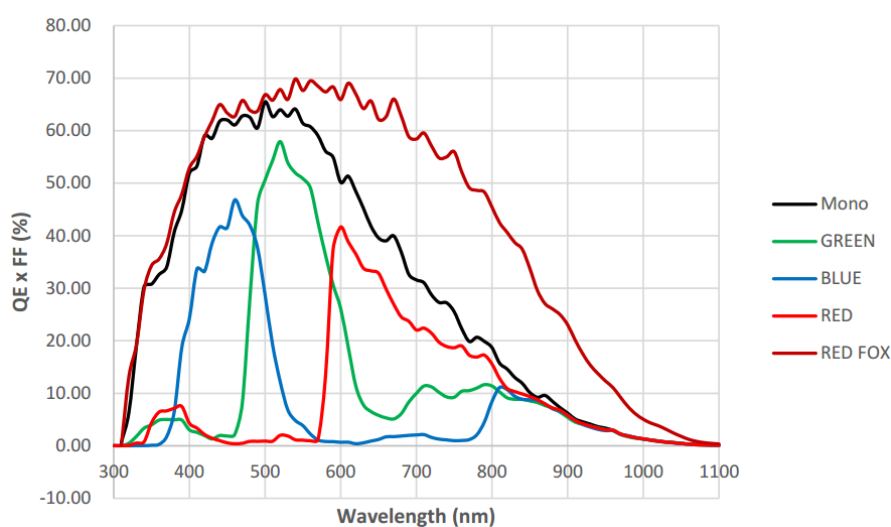
图 4-33 ME2P-2621-15U3M/C \ ME2P-2622-15U3M/C SENSOR 响应曲线
