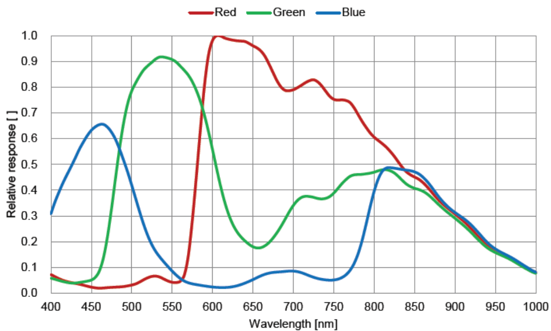
图 4-5 MER2-160-227U3C(-L) SENSOR 响应曲线
