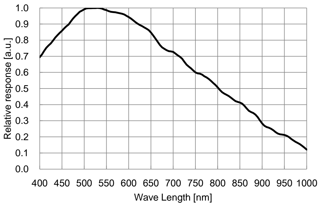
图 4-39 ME2L-505-36U3M(-L) SENSOR 响应曲线
