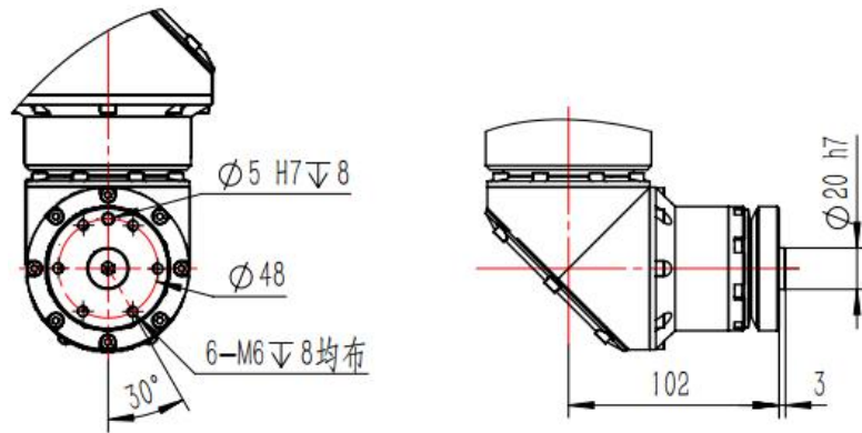
图 3-6 末端负载安装法兰尺寸
