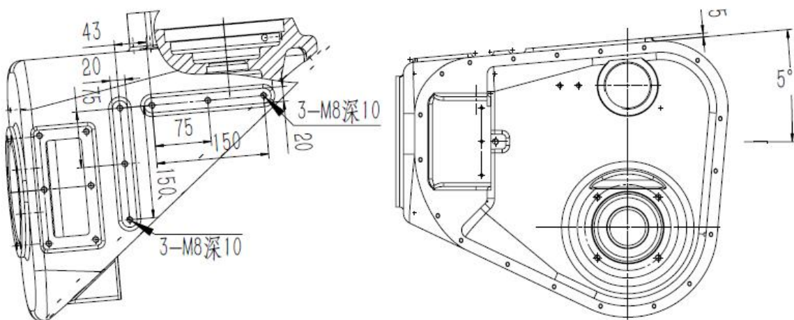
图 3-8 电机座上安装外部件尺寸图
