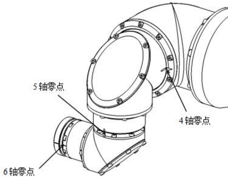
图 4-7 机器人零点位置图
