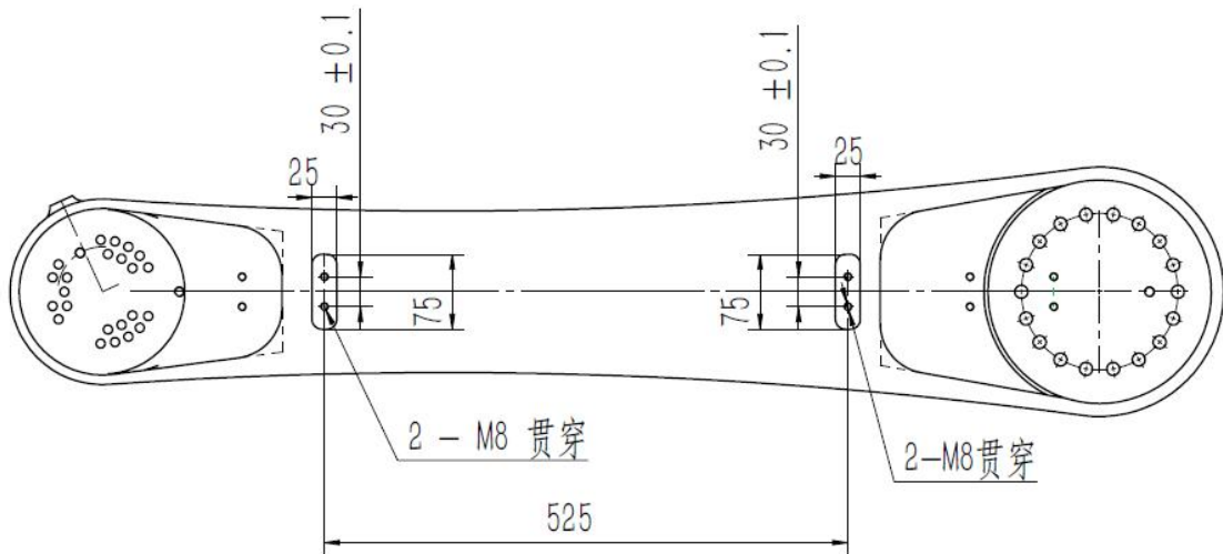
图 3-7 大臂上安装外部件尺寸图
