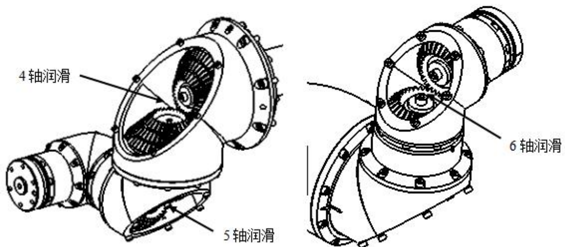
图 4-5 更换润滑油，手腕部分
