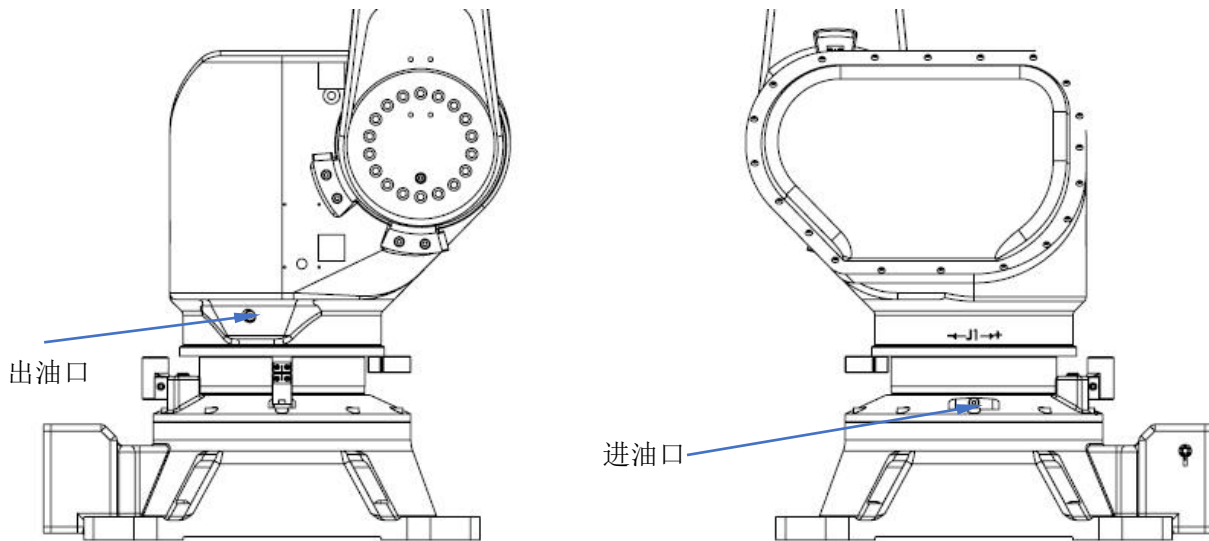
图 4-1 更换润滑油，J1 轴减速机
