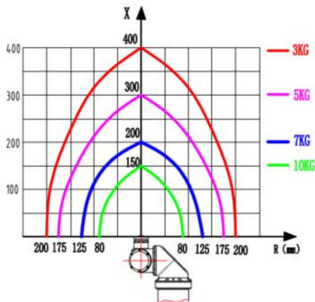
图2-6 GR680手腕轴扭矩图
