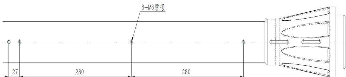
图 3-9 小臂杆上安装外部件尺寸图
