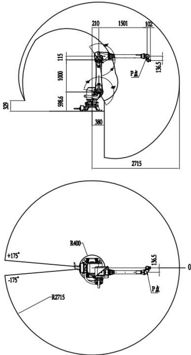
图 2-5 机器人运动范围图
