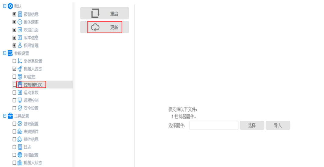
图 3.37 更新固件
