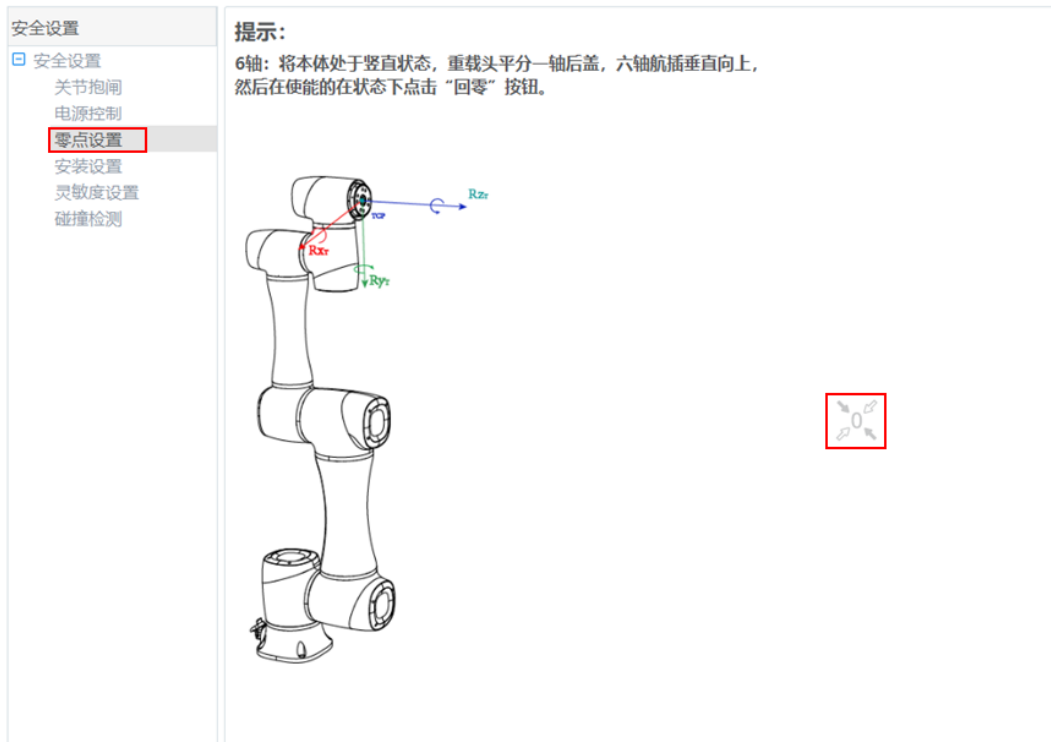
图 3.47 回零
