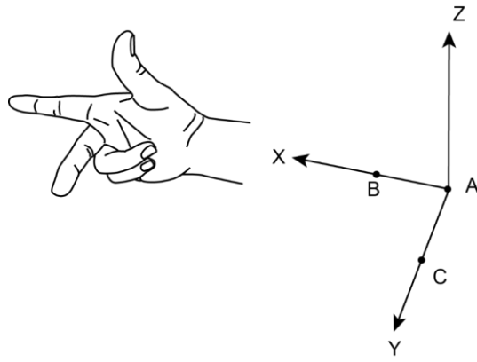
图 3.29 三点示教法
